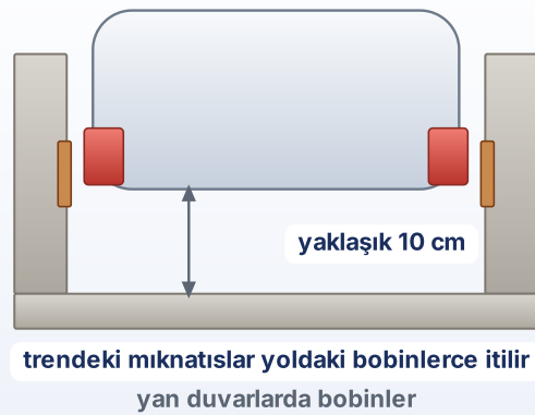
Kaynak 2 · iterek kaldıran sistem
