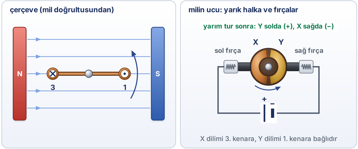
Ş.6 · solda çerçeve, sağda yarık halka ve fırçalar · ikisine de mil doğrultusundan bakılmıştır
