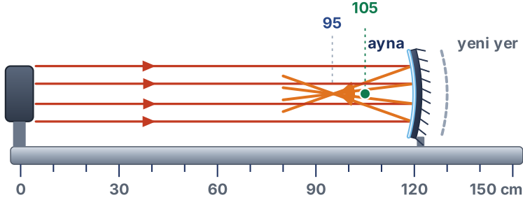
optik tezgâh · aynanın ilk ve yeni yeri
