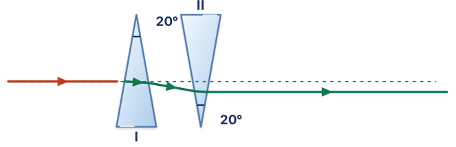
Ş.13 · iki ince prizma · II, I'in ters çevrilmiş hâlidir
