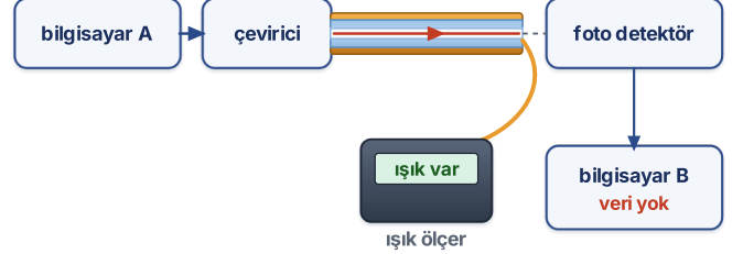
Ş.4 · hattın iki ucu · kablunun ucu ışık ölçere bağlanmış
