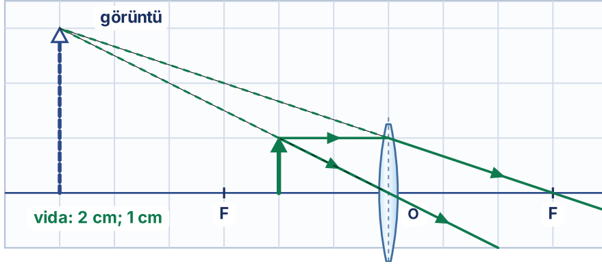
Ş.6 · büyüteç, f = 3 cm, ve saatçinin gördüğü görüntü · 1 kare = 1 cm
