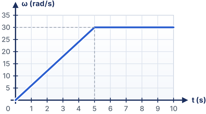
Ş.4 · mıknatıs çubuğun açısal hız–zaman grafiği
