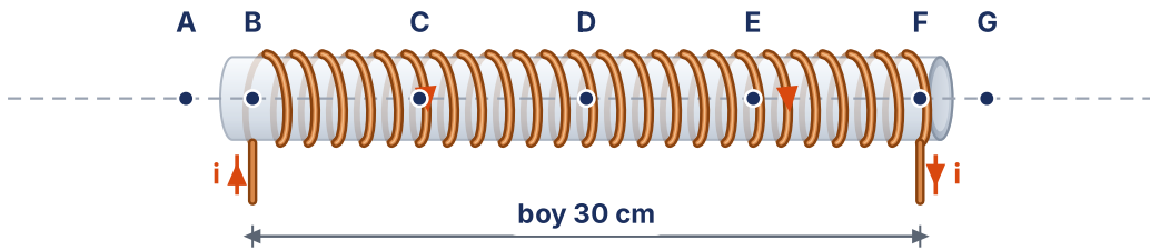
Ş.7 · eksen üzerindeki yedi ölçüm noktası · makaranın N ucu sağdadır
