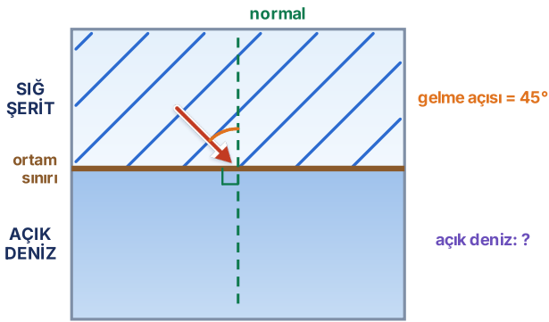
Üstten görünüm - dalga kıyıdan açığa yöneliyor
