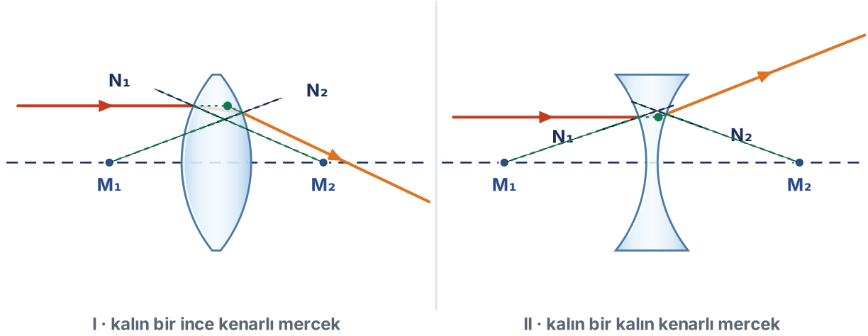
Ş.4 · kalın iki mercekte bir ışının iki yüzeydeki kırılması ( M_1 solda, M_2 sağda)
