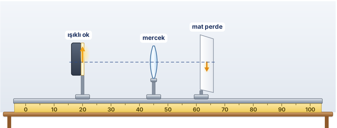
Ş.F1 · ok, mercek ve perde aynı eksende · mercek sabit, ok ve perde kaydırılır
