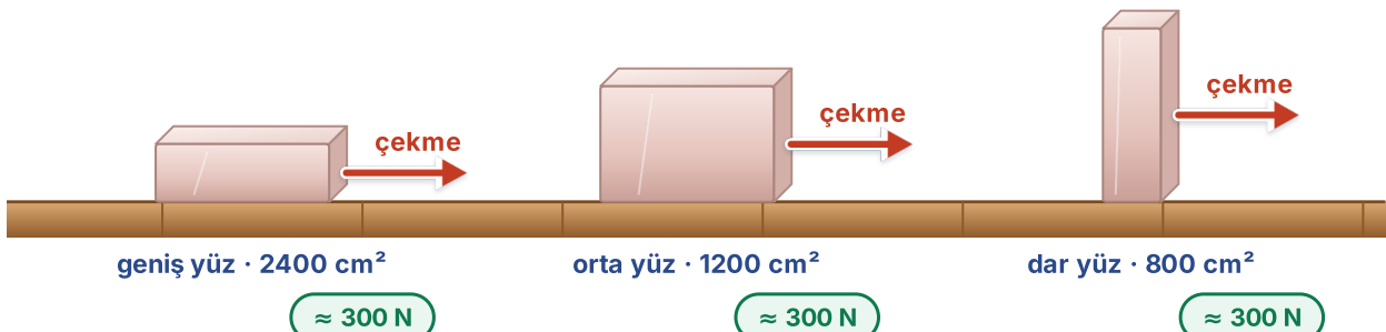
Ş.4 · aynı bloğun üç ayrı yüzü · ağırlık her denemede 1000 N, zemin ahşap kalas
