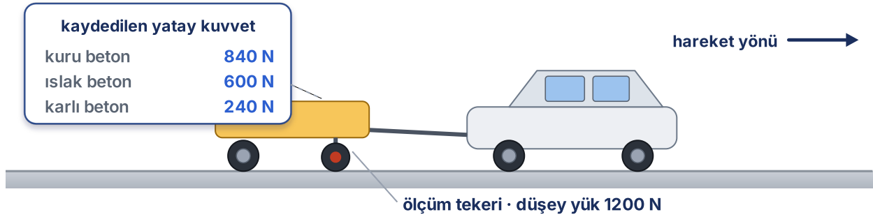
Ş.11 · sürtünme ölçer römork ve ölçüm tekeri · teker dönerken zemine göre kayar
