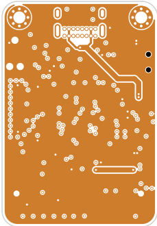
IN2.CU SIGNAL
