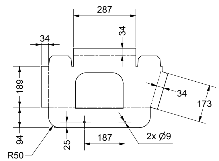
Flat Pattern ( 1 : 10 )
