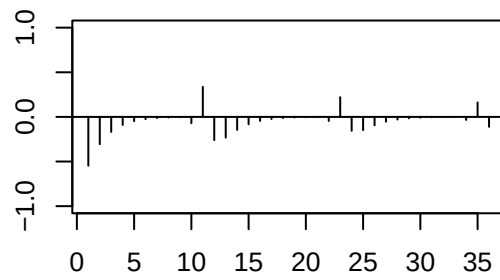
PACF Teoric
