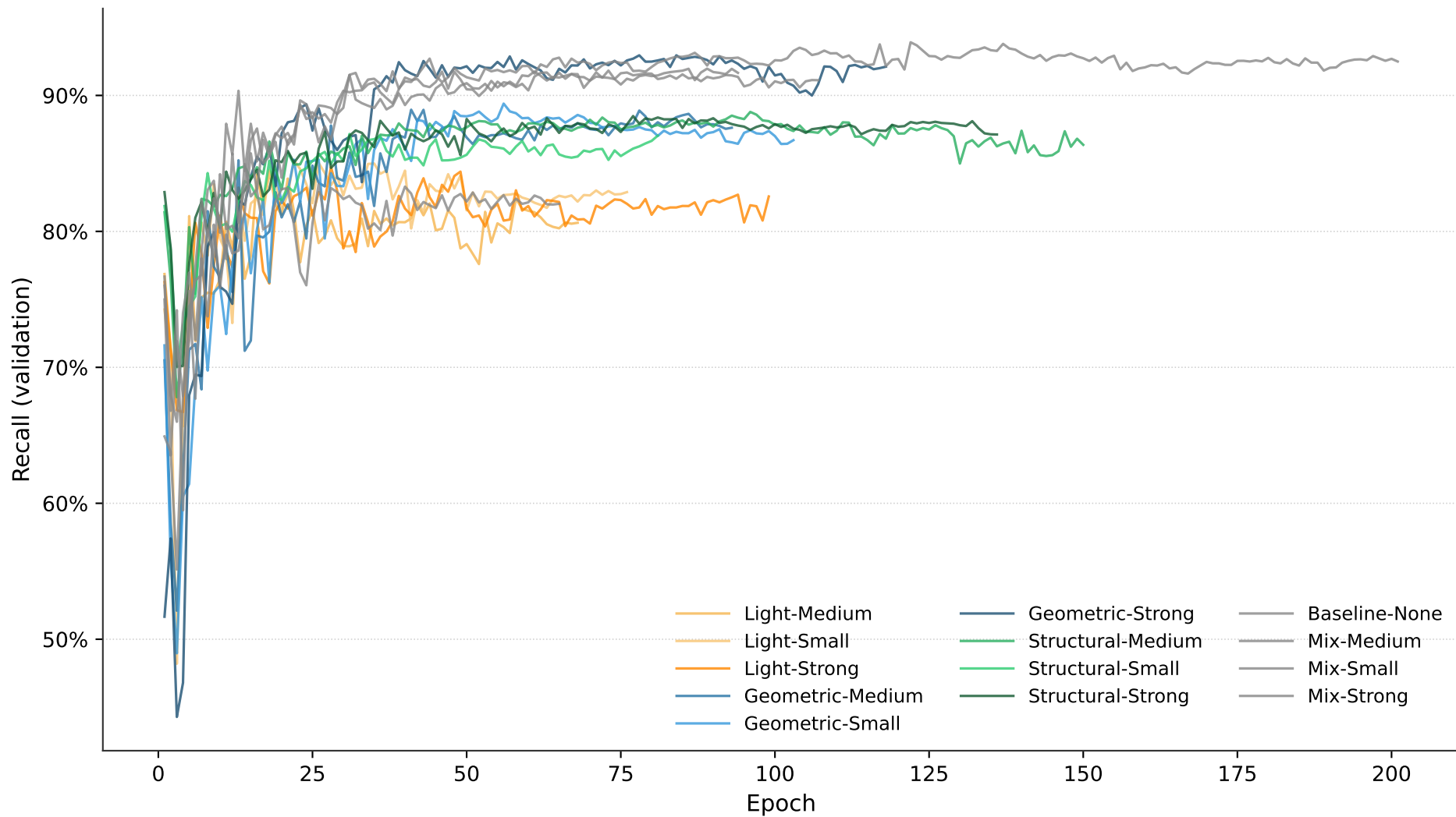
Évolution du Recall sur le validation set
