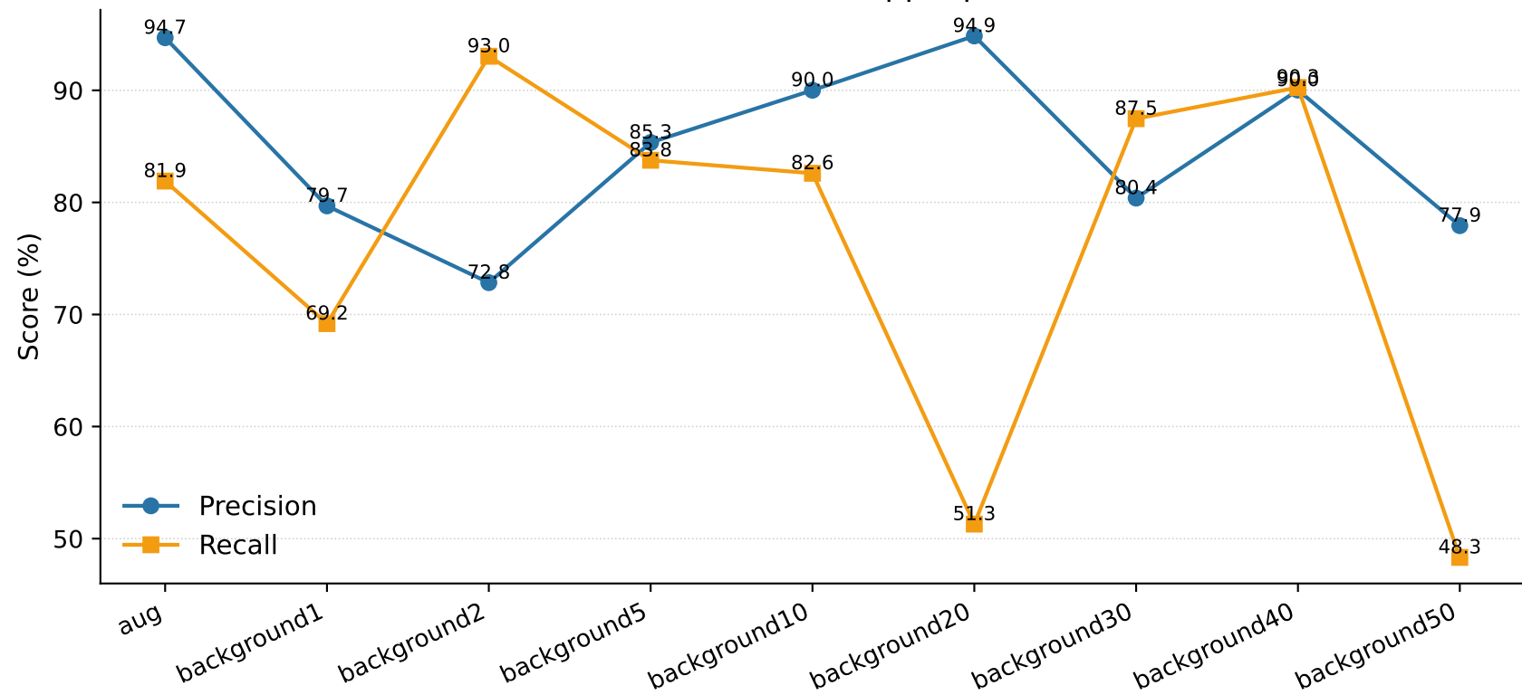
dmcode — Précision et rappel par modèle
