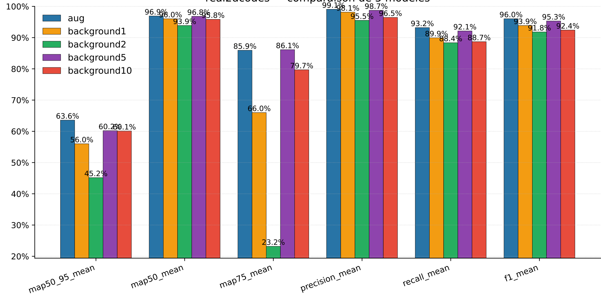
real2dcodes — comparaison de 5 modèles
