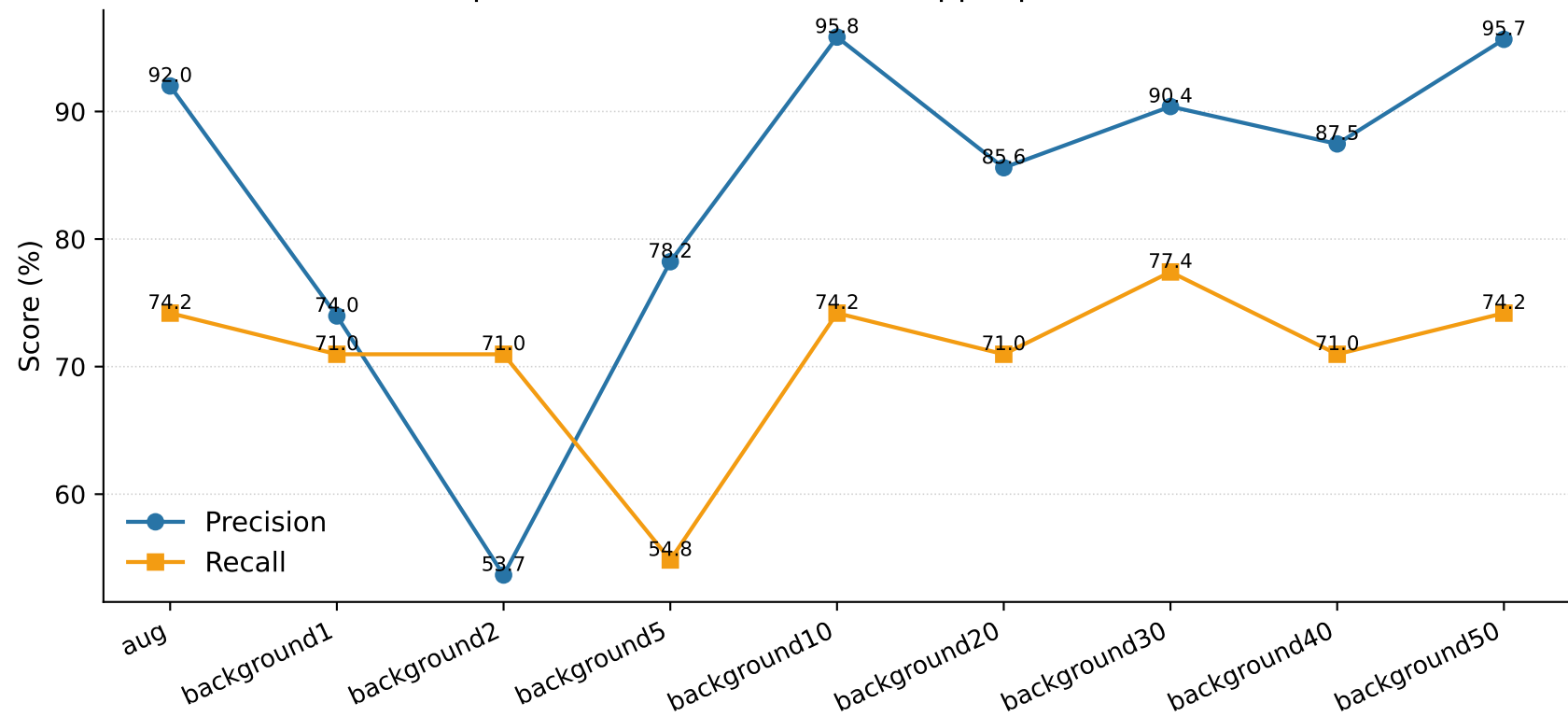
pcbdataset — Précision et rappel par modèle
