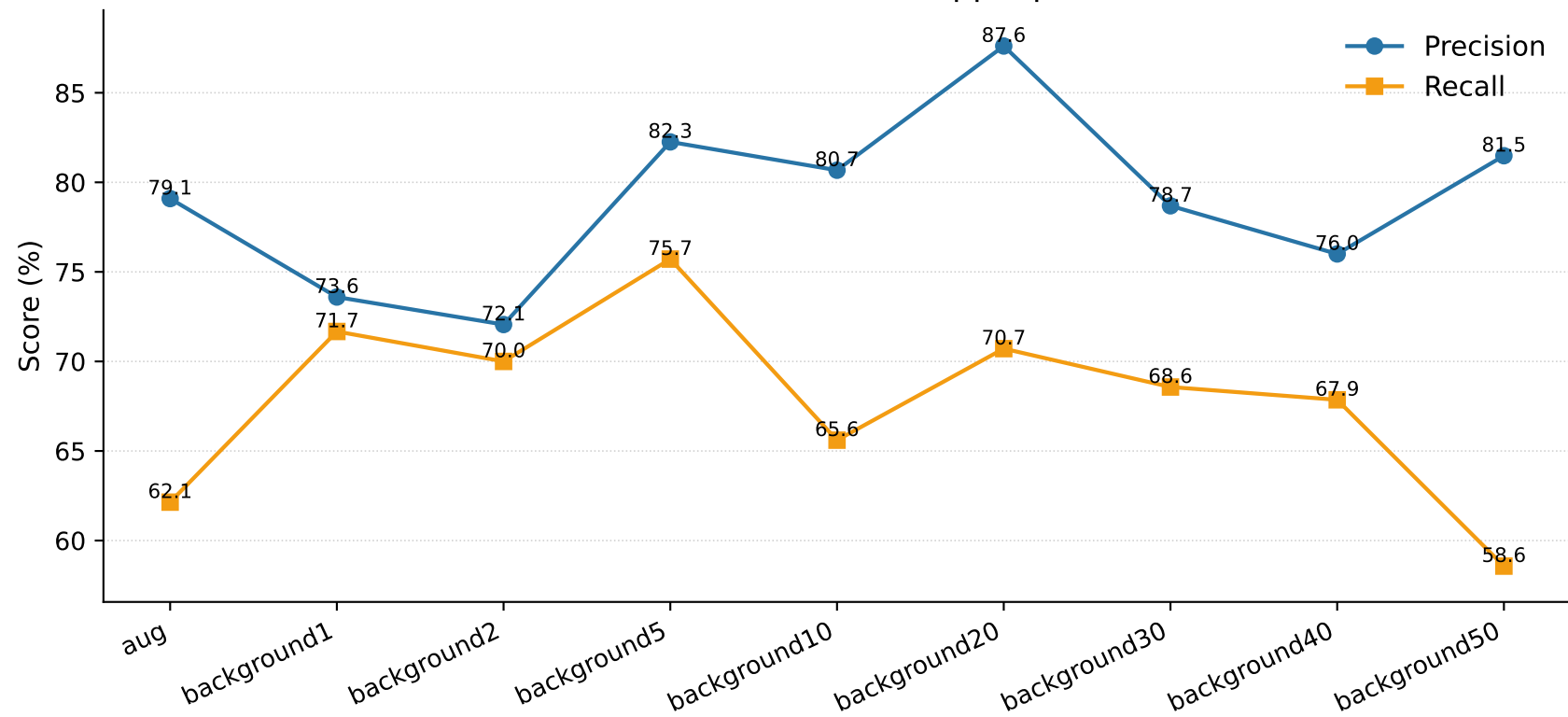
datamatrixfit — Précision et rappel par modèle
