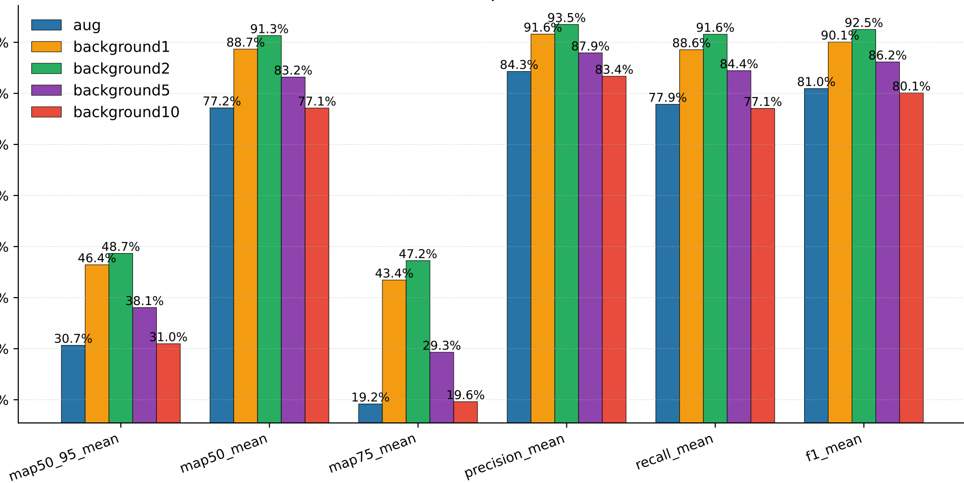
datamatrix140 — comparaison de 5 modèles
