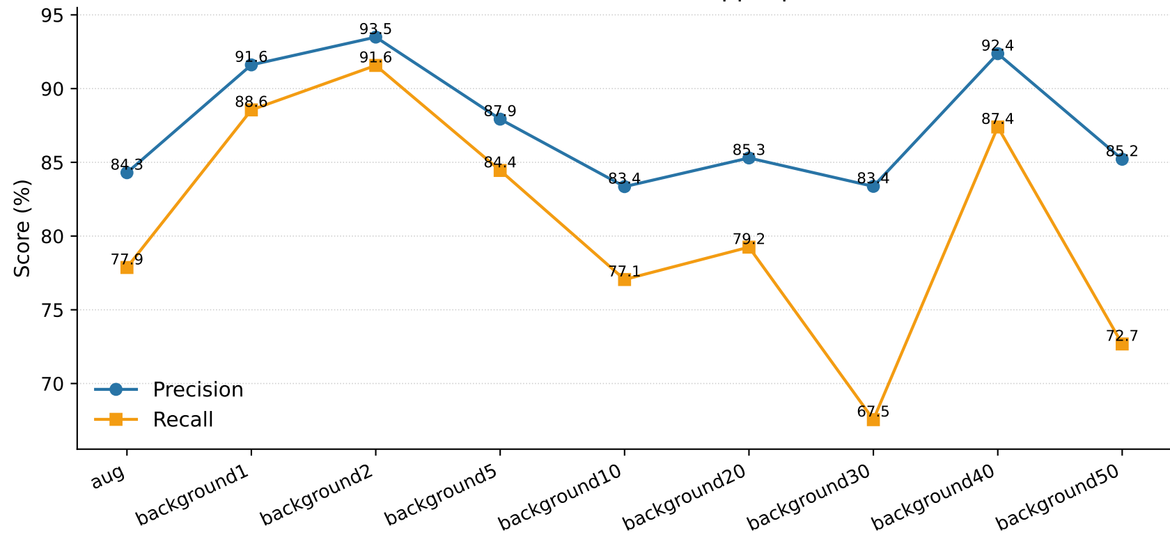
datamatrix140 — Précision et rappel par modèle
