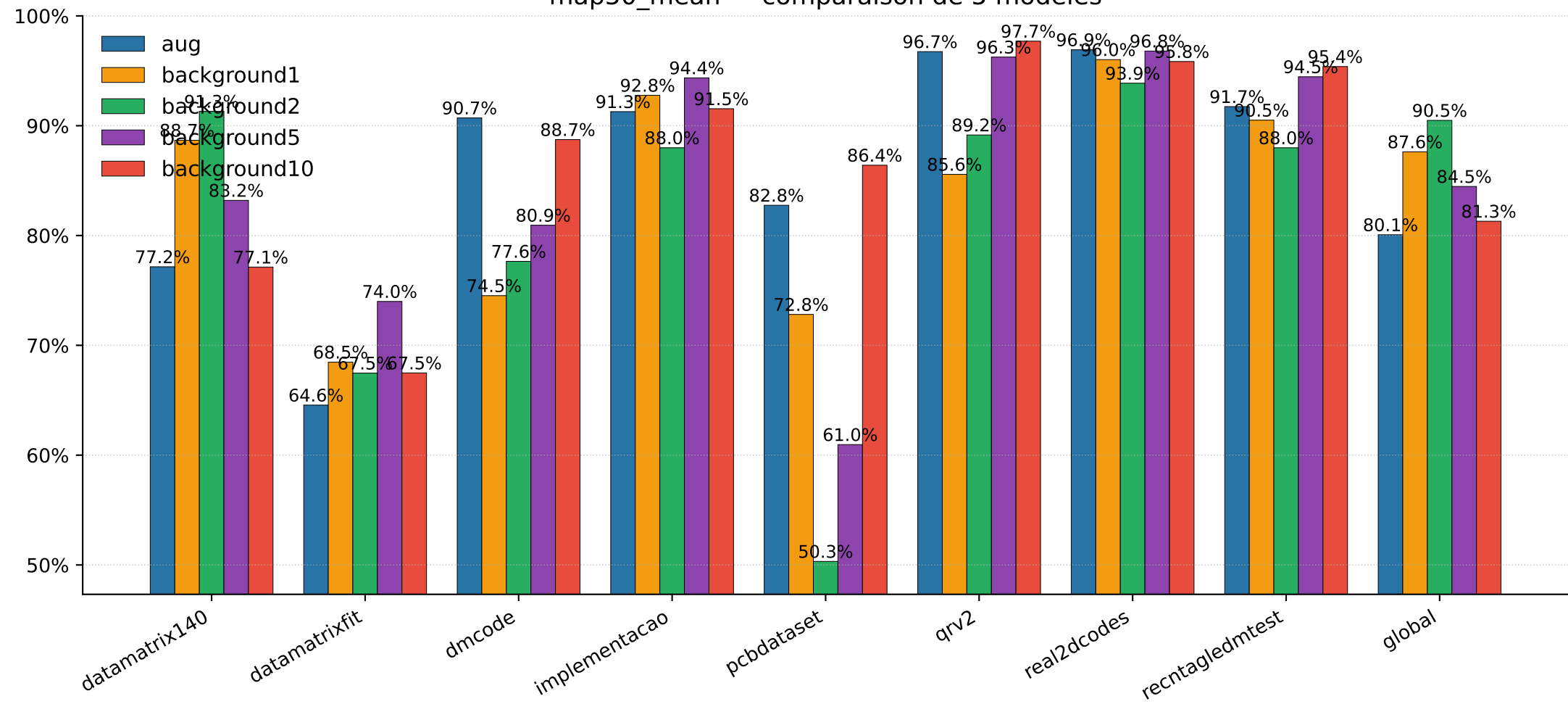
map50_mean — comparaison de 5 modèles
