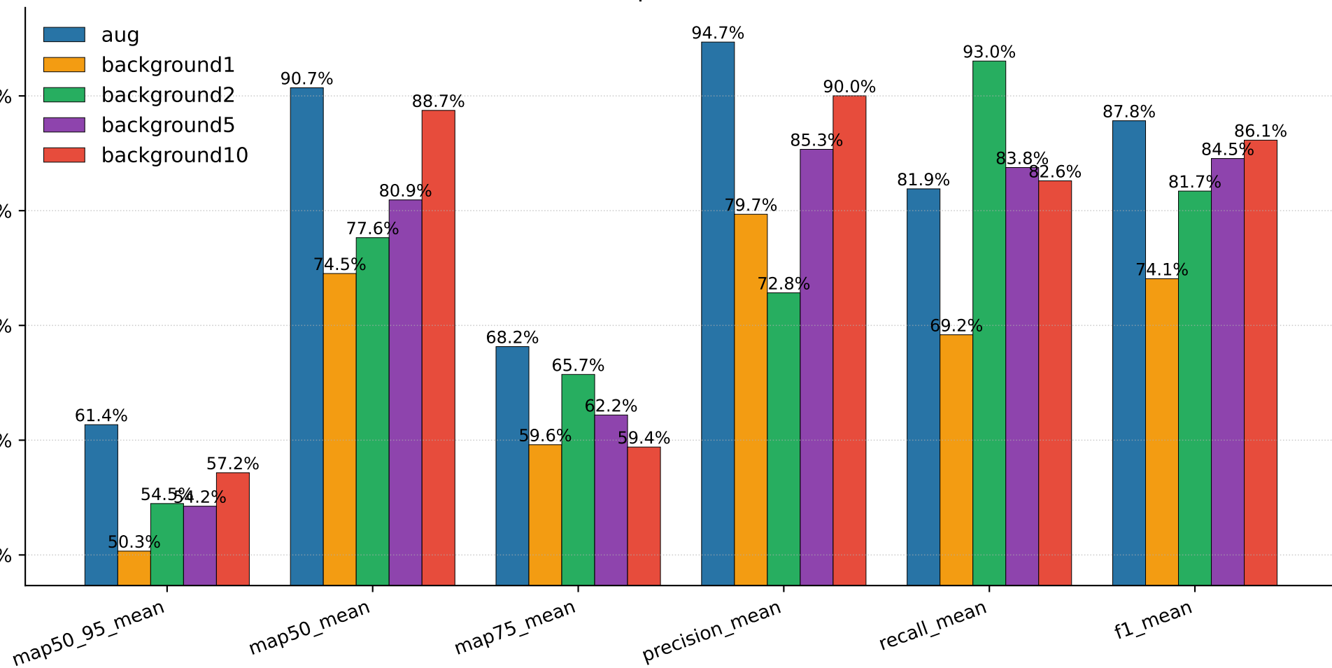
dmcode — comparaison de 5 modèles
