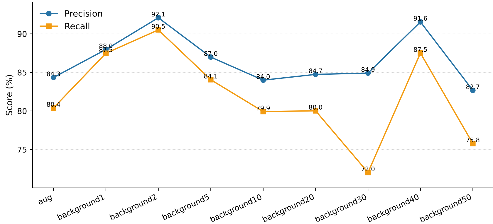
global — Précision et rappel par modèle
