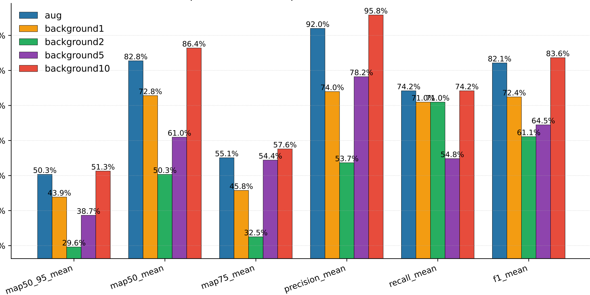
pcbdataset — comparaison de 5 modèles
