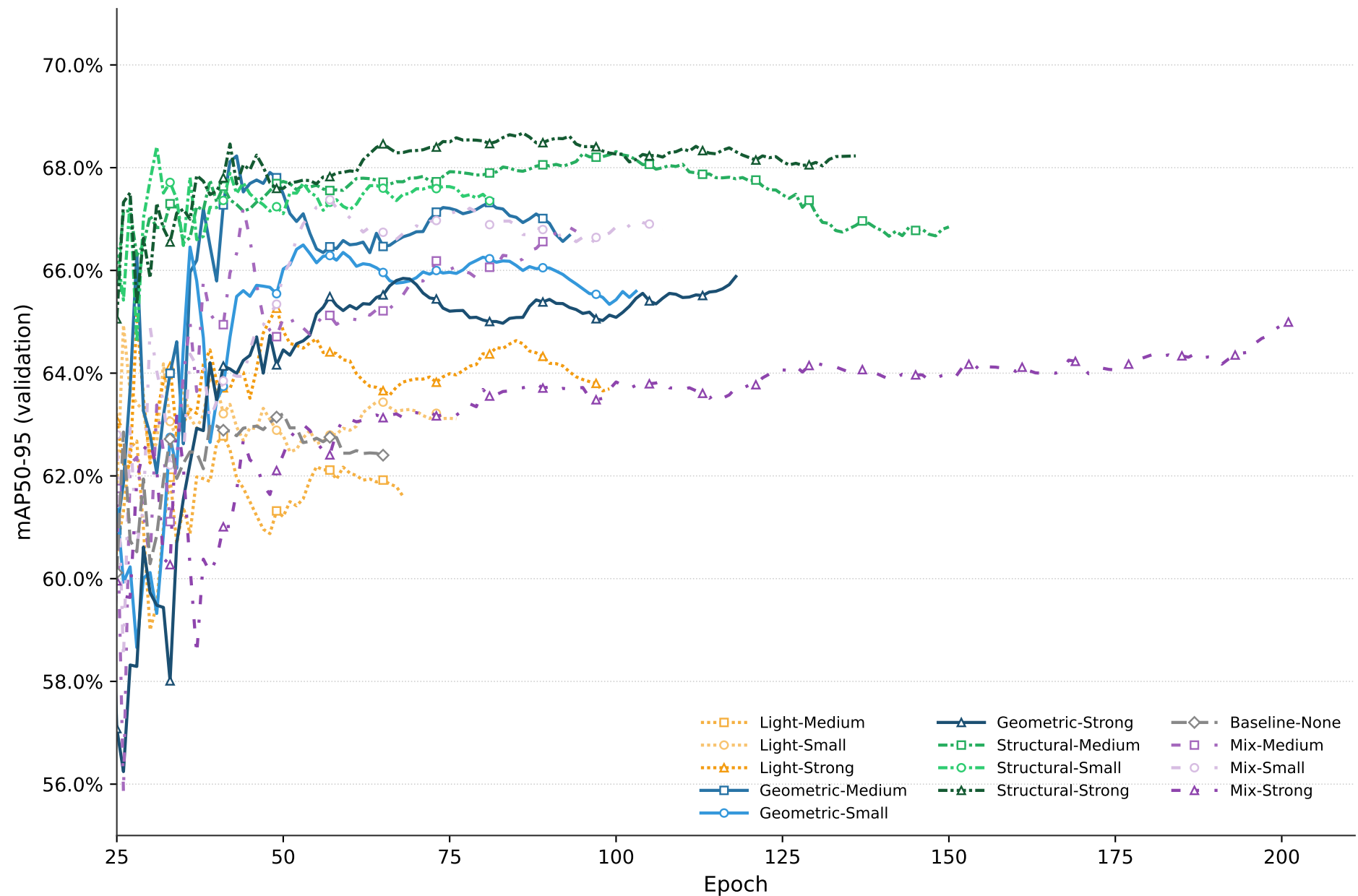
Évolution du mAP50-95 sur le validation set
