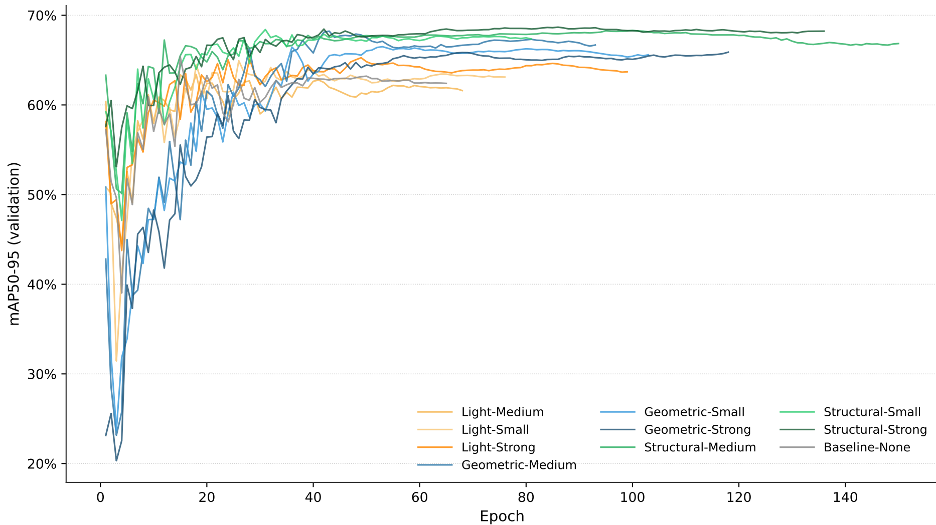
Évolution du mAP50-95 sur le validation set
