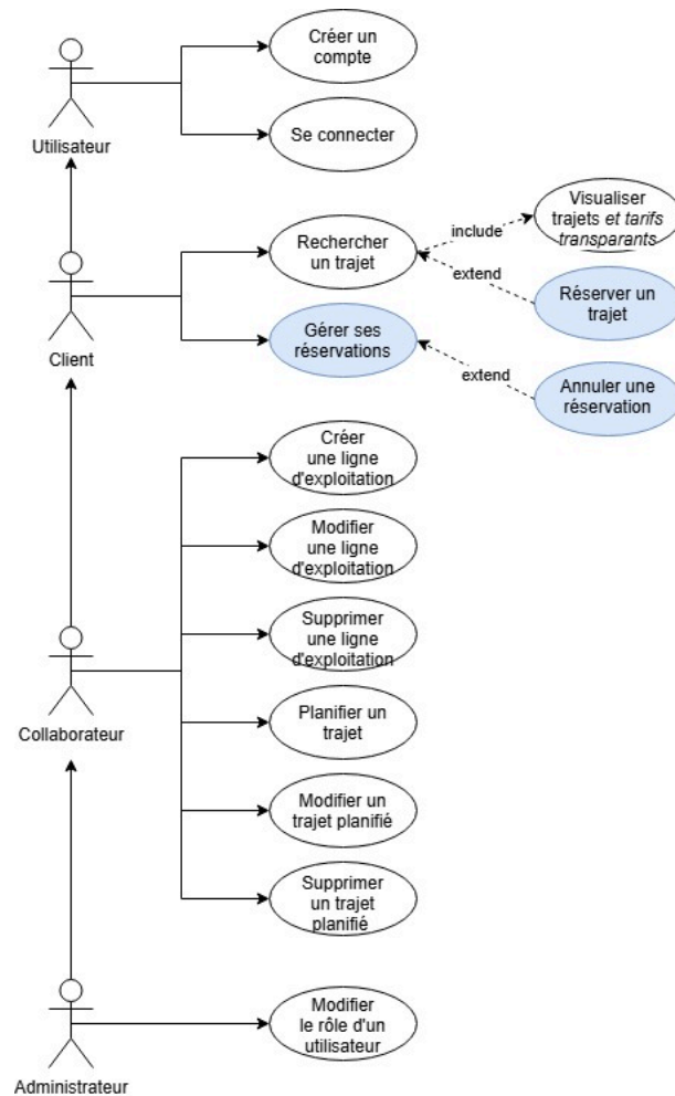
Figure 2: Cas d'utilisation
