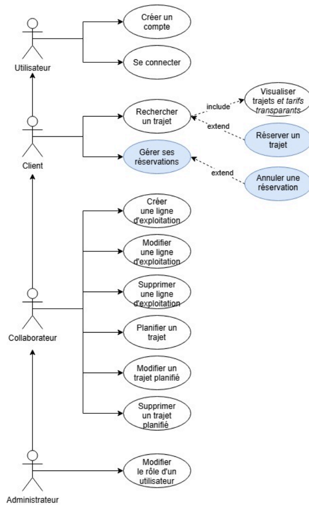
Figure 2: Cas d'utilisation
