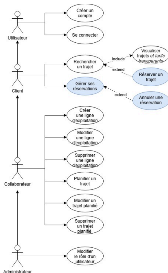
Figure 2: Cas d'utilisation
