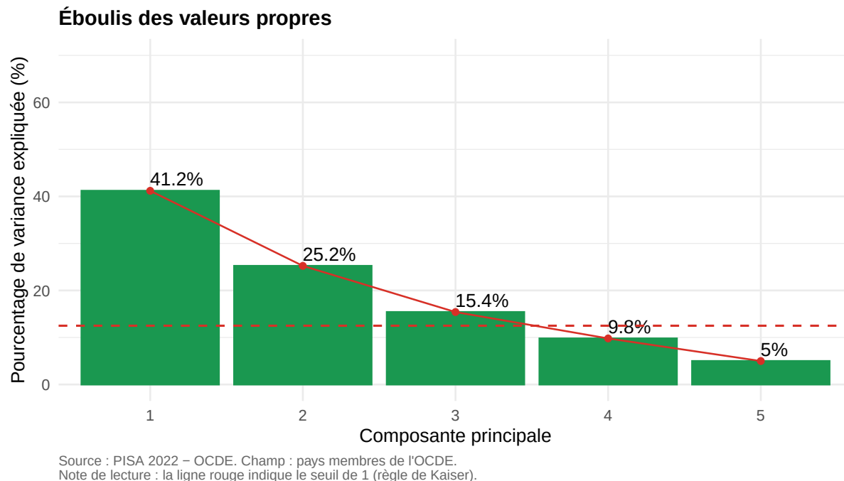
FIGURE 20 : Éboulis des valeurs propres
