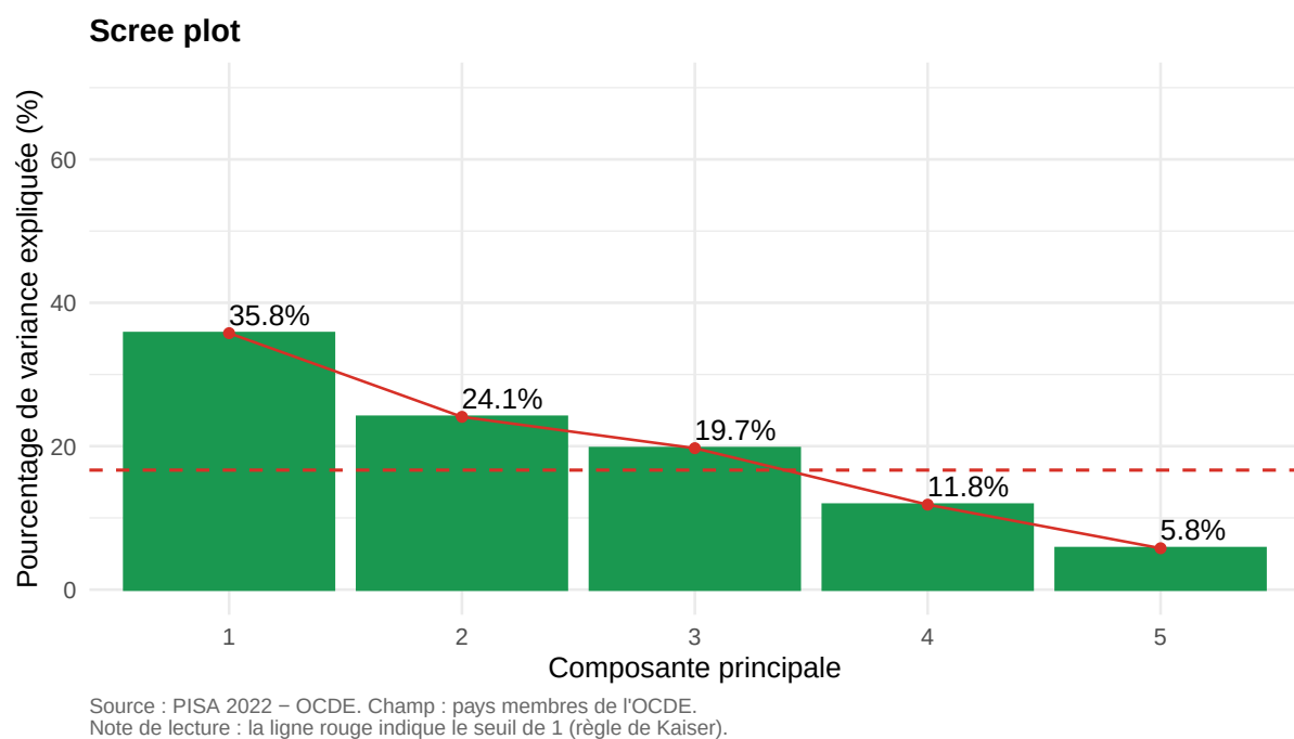
FIGURE 17 : Éboulis des valeurs propres
