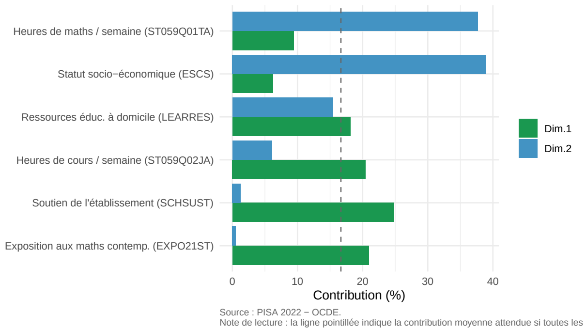
FIGURE 20 : Contribution des variables aux axes 1 et 2
