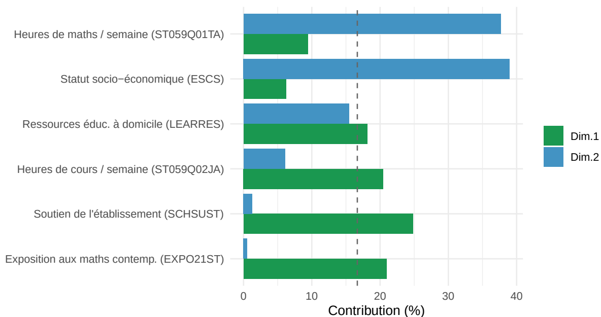
FIGURE 20 : Contribution des variables aux axes 1 et 2
