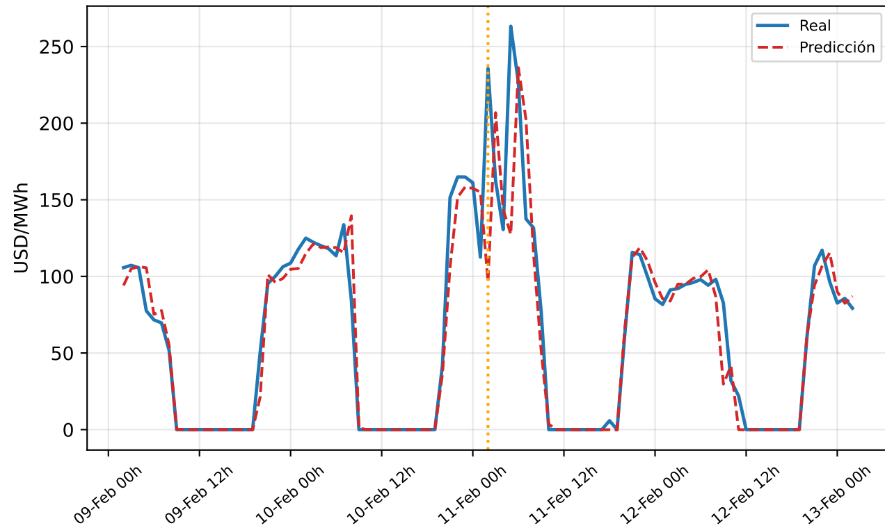
#5: 2025-02-11 02:00:00 — Desfase de fase (error=139.2)
