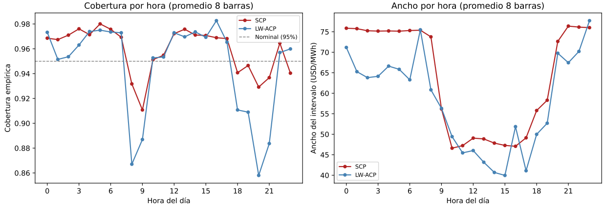
Figura 4.3: Cobertura empírica (izquierda) y ancho medio del intervalo (derecha) por hora del día, Split CP vs. LW-ACP, promediado sobre las ocho barras. LW-ACP es más angosto que Split CP casi todo el día, pero su cobertura cae marcadamente por debajo del nominal en las horas de transición solar (7–9h, 19–21h).
