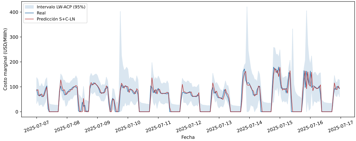
Figura 4.2: Ejemplo de intervalo de predicción LW-ACP (95 % nominal) para Atacama, 10 días del conjunto de prueba (7–17 de julio de 2025). El intervalo se angosta en las horas de precio cero (madrugada, sobreoferta solar) y se ensancha ante los spikes de precio, como el del 9 de julio.
