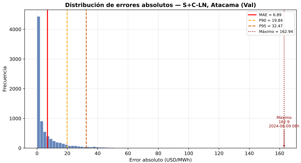
Figura 4.4: Distribución de errores absolutos del TFT_{LN} (S+C) en el conjunto de validación para la barra Atacama ( n = 8\,298 observaciones). Las líneas verticales indican el MAE (rojo), el percentil 90 (naranja claro), el percentil 95 (naranja oscuro) y el error máximo (granate, punteado), este último señalado además con una flecha dado lo alejado que queda del grueso de la distribución.
