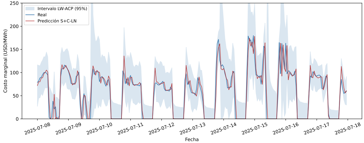
Figura 4.2: Ejemplo de intervalo de predicción LW-ACP (95 % nominal) para Atacama, 10 días del conjunto de prueba (8–18 de julio de 2025). El eje vertical se acota en 250 USD/MWh por legibilidad: el intervalo supera ese límite en algunas horas puntuales (por ejemplo, en torno al 9–10 de julio), consistente con que \alpha_t se ensancha tras un error de cobertura reciente (Sección 3.7.3). El intervalo se angosta en las horas de precio cero (madrugada, sobreoferta solar) y captura correctamente los spikes de precio de mediados de mes (14–16 de julio).
