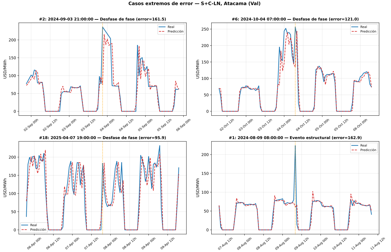
Figura 4.5: Casos extremos de error del TFT_{LN} (S+C) para la barra Atacama en validación. Cada panel muestra una ventana de \pm 48h alrededor del instante de error máximo (línea vertical punteada naranja). La curva azul corresponde al CMg real y la curva roja punteada a la predicción.
