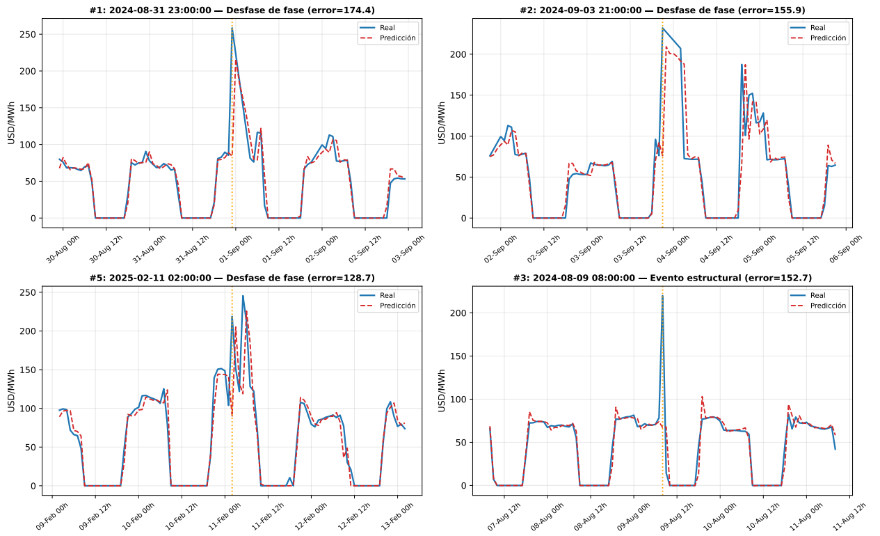
Figura A.3: Casos extremos de error del T TFT LN (S+C), Crucero.
