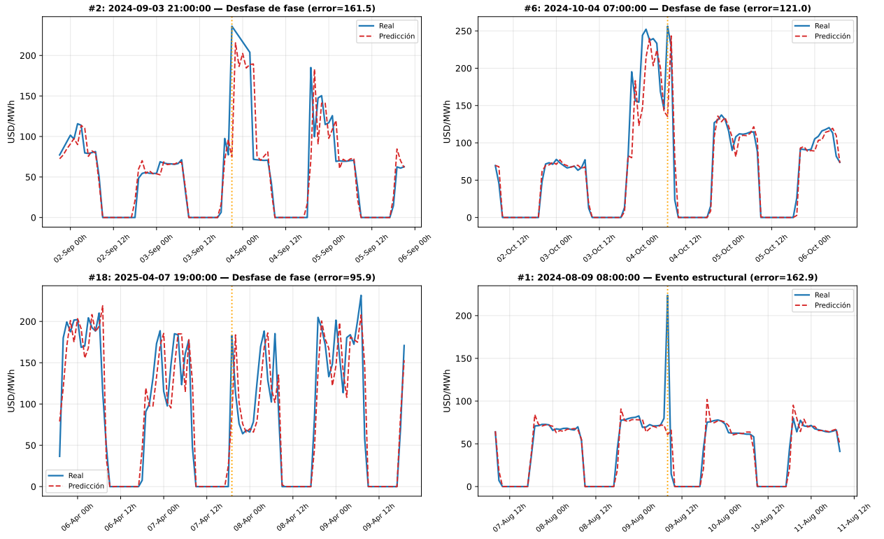
Figura 4.3: Casos extremos de error del TFT_{LN} (S+C) para la barra Atacama en validación. Cada panel muestra una ventana de \pm 48 h alrededor del instante de error máximo (línea vertical punteada naranja). La curva azul corresponde al CMg real y la curva roja punteada a la predicción.
