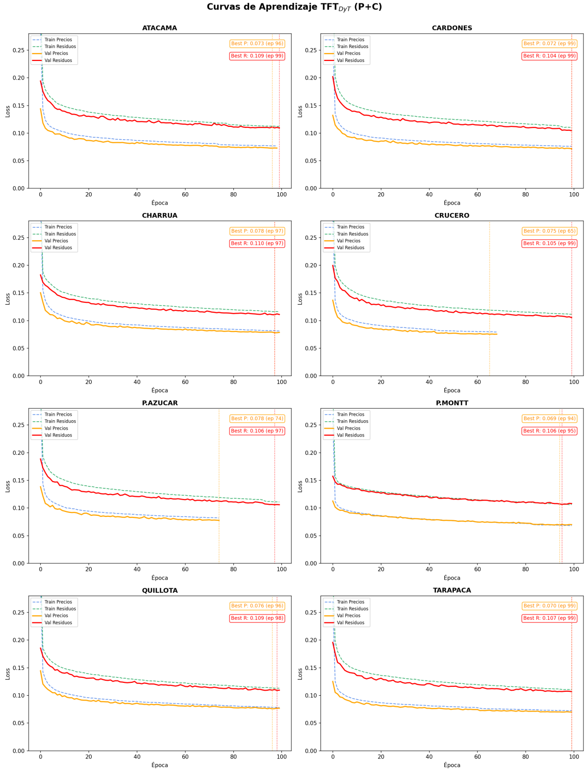
Figura 3.5: Curvas de aprendizaje del TFT con DyT para las ocho barras del SEN. Se muestran la pérdida (MAE) de entrenamiento y validación para los modelos de precios y residuos. Las líneas verticales indican la época de mejor desempeño en validación.
