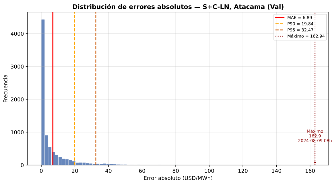
Figura 4.4: Distribución de errores absolutos del \text{TFT}_{\text{LN}} (S+C) en el conjunto de validación para la barra Atacama ( n = 8\,298 observaciones). Las líneas verticales indican el MAE (rojo), el percentil 90 (naranja claro), el percentil 95 (naranja oscuro) y el error máximo (granate, punteado), este último señalado además con una flecha dado lo alejado que queda del grueso de la distribución.
