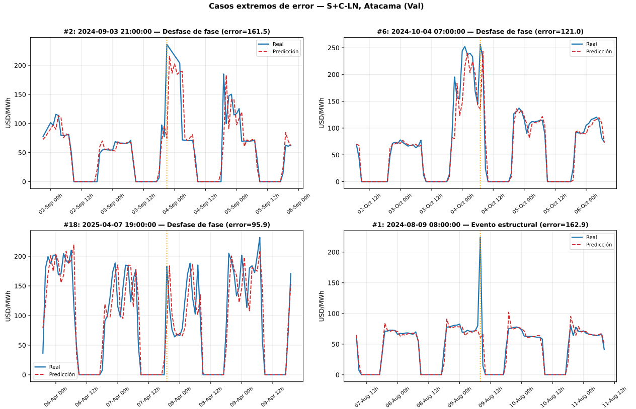
Figura 4.5: Casos extremos de error del \text{TFT}_{\text{LN}}(\text{S}+\text{C}) para la barra Atacama en validación. Cada panel muestra una ventana de \pm 48 h alrededor del instante de error máximo (línea vertical punteada naranja). La curva azul corresponde al CMg real y la curva roja punteada a la predicción.
