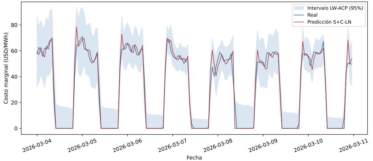
Figura 4.2: Ejemplo de intervalo de predicción LW-ACP (95 % nominal) para Atacama, 4–11 de marzo de 2026. El intervalo se angosta en las horas de precio cero (sobreoferta solar) y se ensancha en las horas de transición, siguiendo de cerca el ciclo diario del precio.
