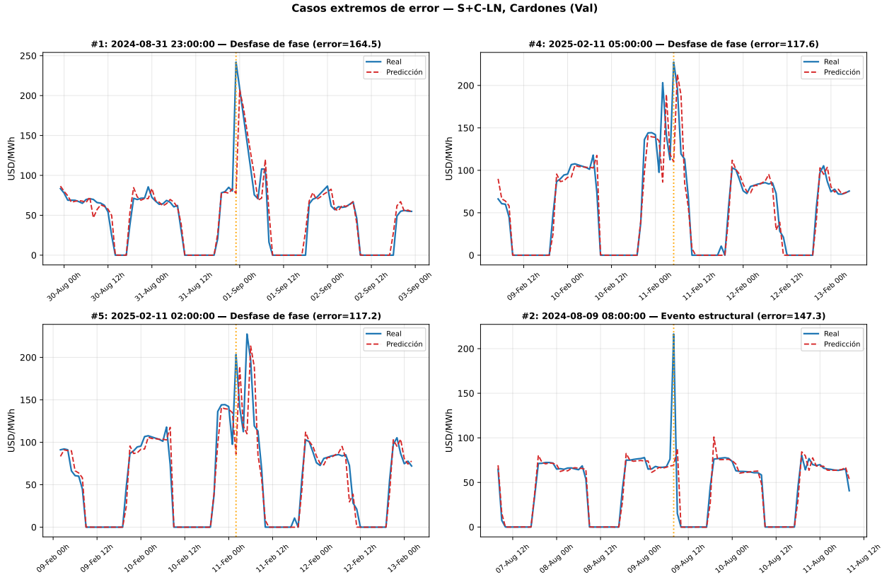
Figura A.1: Casos extremos de error del TFT_{LN} (S+C), Cardones.
