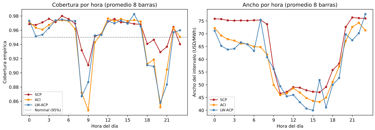
Figura 4.3: Cobertura empírica (izquierda) y ancho medio del intervalo (derecha) por hora del día, Split CP vs. ACP vs. LW-ACP, promediado sobre las ocho barras. ACP y LW-ACP son más angostos que Split CP casi todo el día, pero ambos –no solo LW-ACP– caen marcadamente por debajo del nominal en las horas de transición solar (7–9h, 19–21h).
