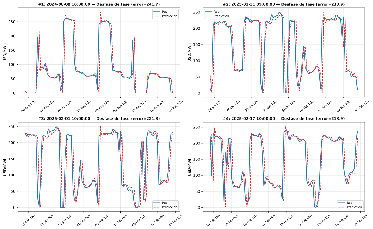
Figura A.5: Casos extremos de error del TTF LN (S+C), Puerto Montt.
