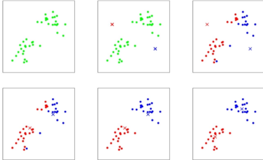
Figura 12.8: K-Means algorithm, retomado de Ng (2023, p 146) [NG]
