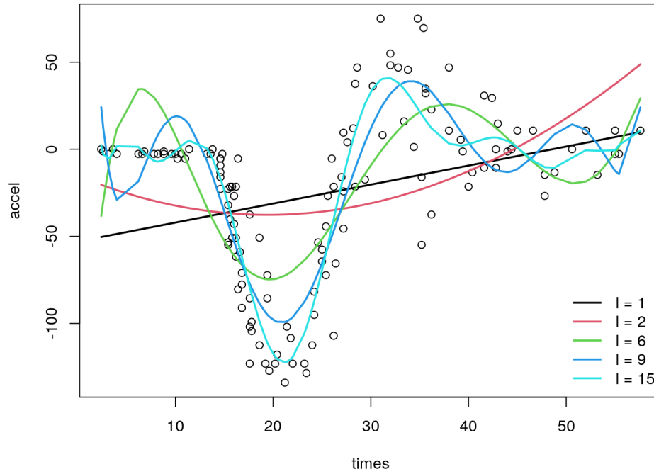
Figura 12.5: Funciones polinomiales, retomado de https://discdown.org/flexregression/smoothreg.html
