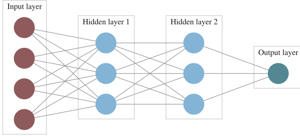
Figura 12.15: Ejemplo de redes neuronales. Retomado de Shmueli et al (2019, 285) [Shm+19]
