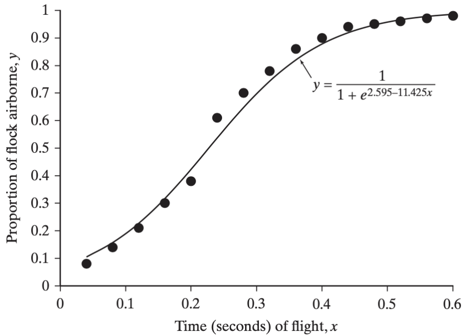
Figura 12.4: Funciones logísticas, Retomado de Larsen y Marx (2012, p. 540) [LARSEN]
