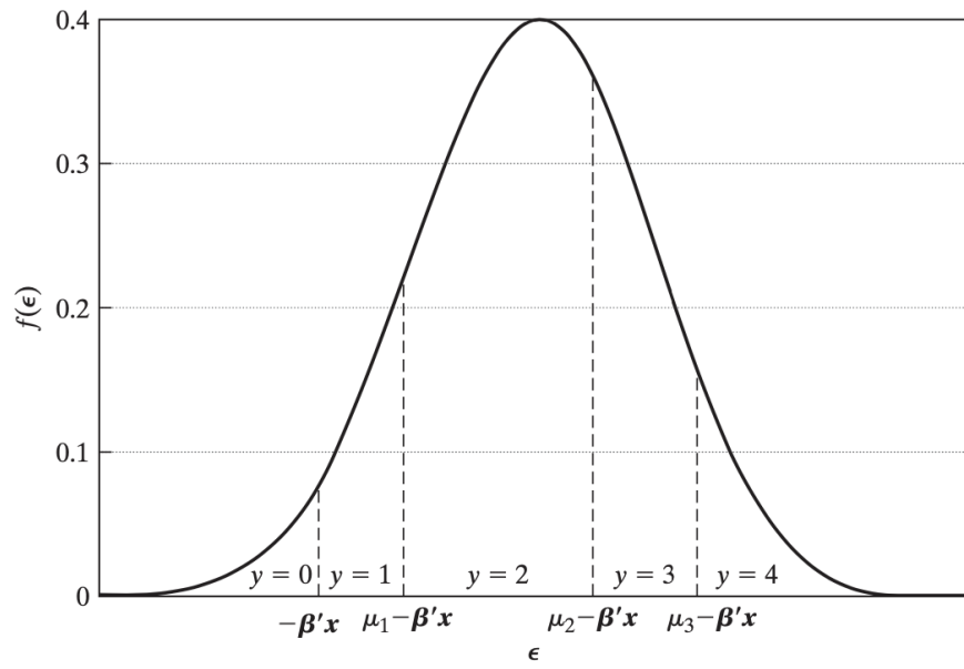
Figura 12.11: Probabilidades en un modelo de respuesta ordenada, considerando J = 4 (retomado de Greene (2012, 788) [Gre12])
