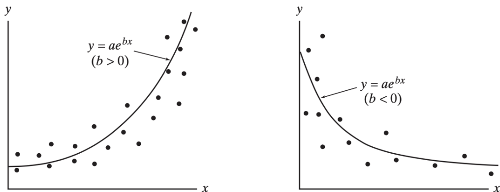
Figura 12.2: Funciones exponenciales, Retomado de Larsen y Marx (2012, p. 532) [LARSEN]
