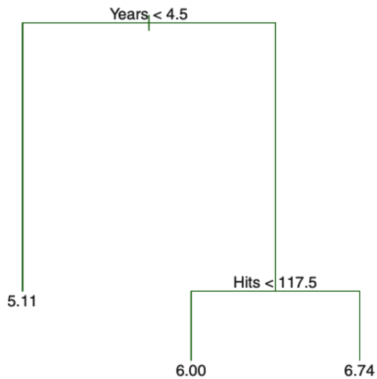
Figura 12.14: Ejemplo de árbol. Retomado de Hastie et al (2017, 304)
