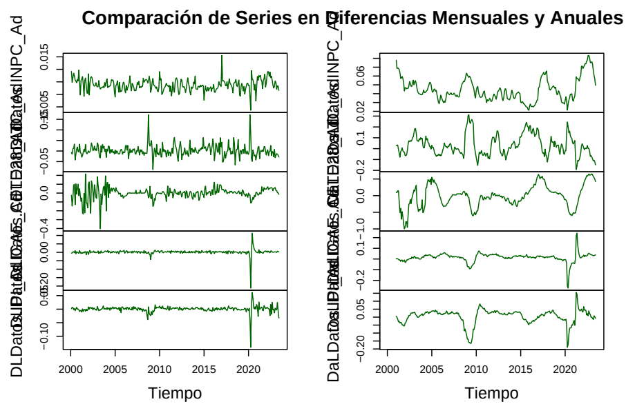
Figura 4.5: Comparación de Series en Diferencias Mensuales y Anuales (Logarítmicas)
