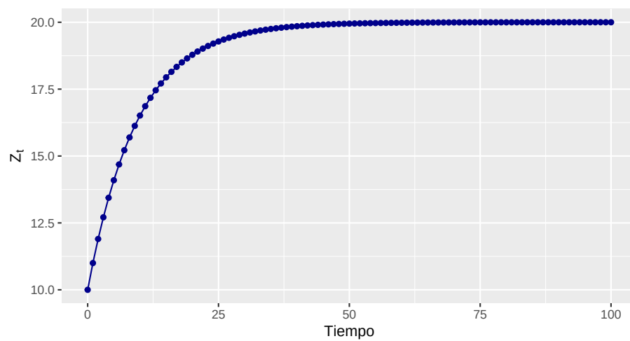
Figura 2.6: Evolución del proceso dado por Z_t = 2 + 0.9Z_{t-1}
