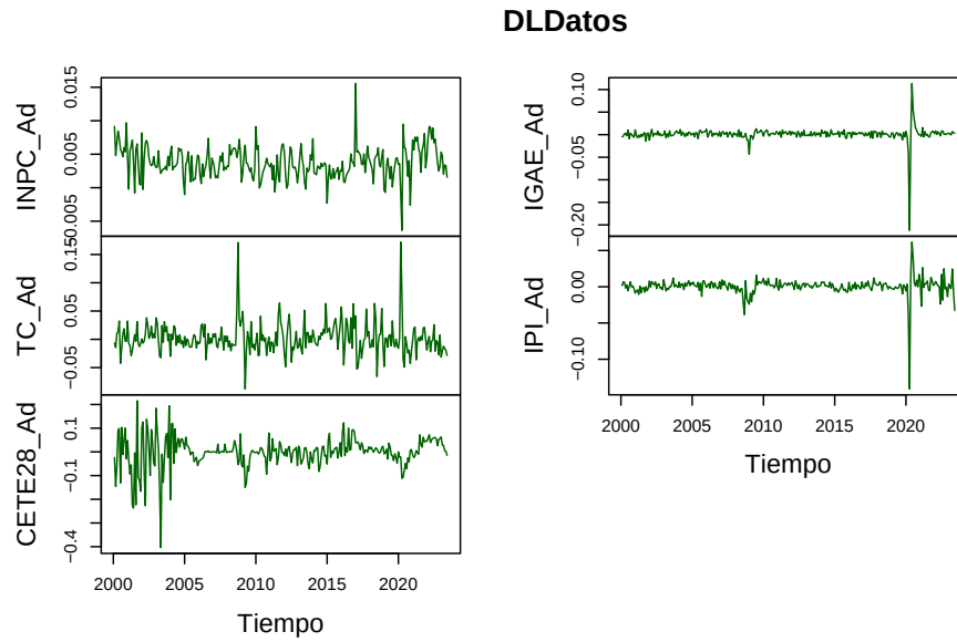
Figura 5.10: Series en Diferencias Logarítmicas para la prueba de Cointegración
