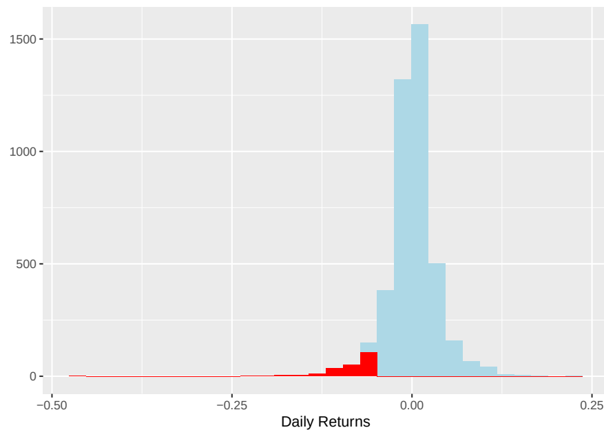
Figura 6.3: Histograma de rendimientos del Bitcoin
