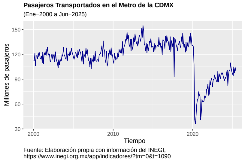
Figura 3.2: Evolución del número de pasajeros en el Metro de la CDMX, enero 2000 a junio 2025
