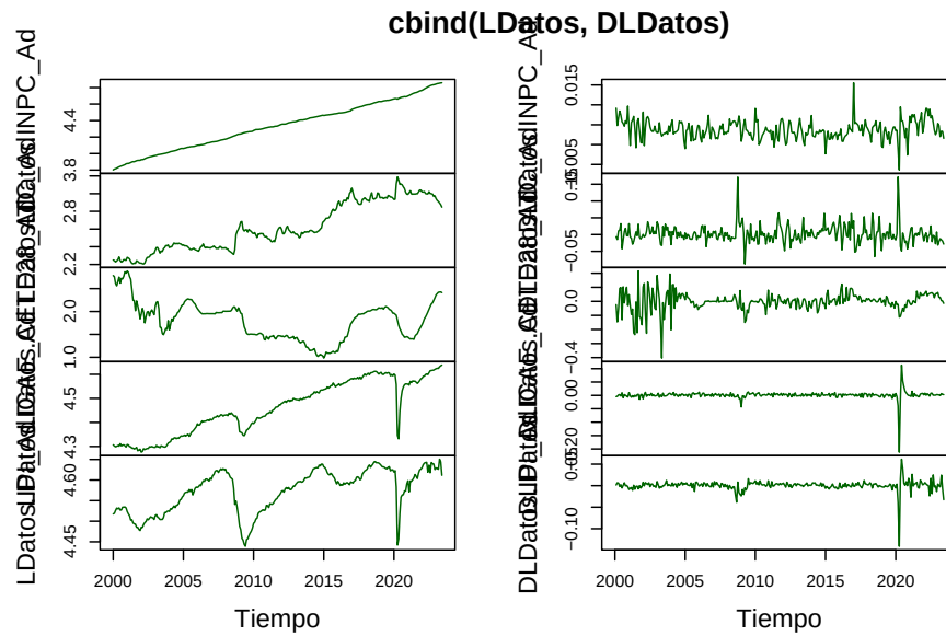
Figura 5.11: Comparación de Series en Diferencias para la prueba de Cointegración
