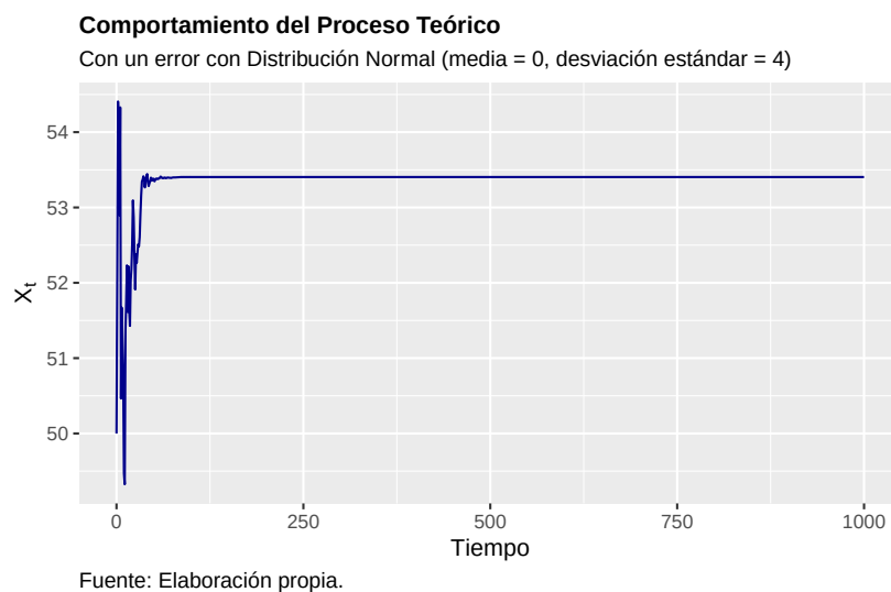
Figura 3.5: Comportamiento del Proceso Teórico
