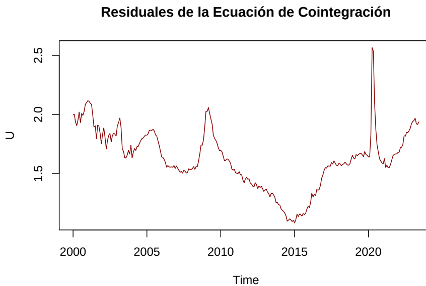
Figura 5.12: Residuales estimados de la ecuación de cointegración
