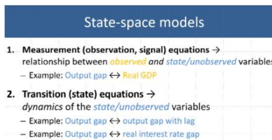
Figura 5.15: State-space models. Recuperado de IMF [-@imf2020].
