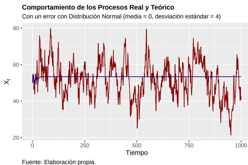
Figura 3.8: Comportamiento de los Procesos Real y Teórico
