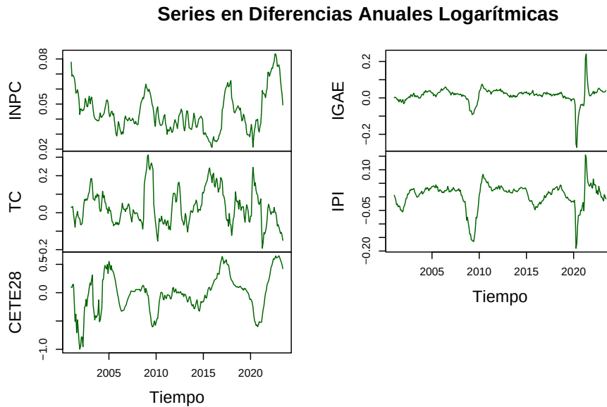
Figura 4.4: Series en Diferencias Anuales Logarítmicas
