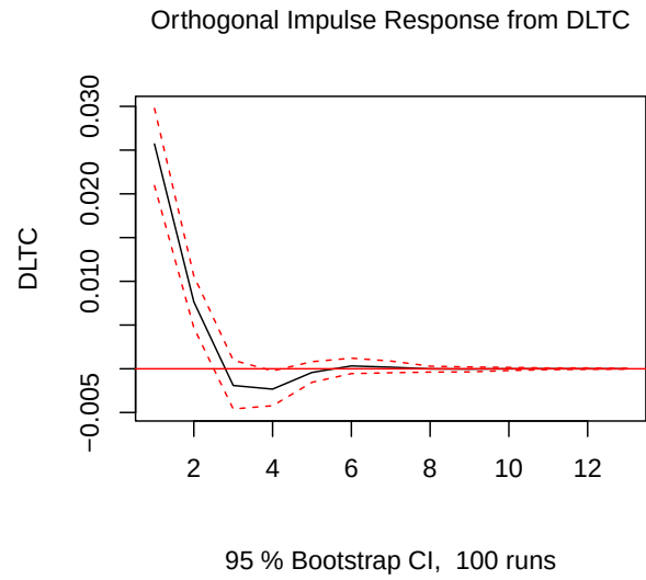
Figura 5.5: Impulso - Respuesta en DLTC_t
