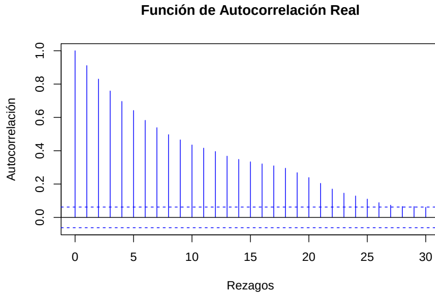
Figura 3.6: Función de Autocorrelación Real
