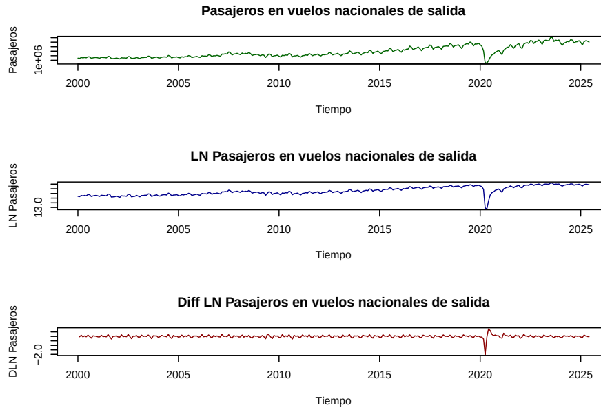
Figura 3.10: Pasajeros en vuelos de salidas nacionales en niveles y en diferencias logarítmicas
