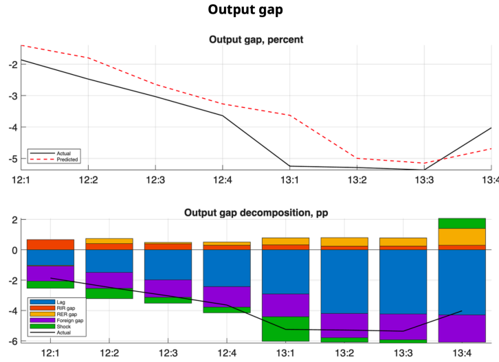
Figura 5.16: Simulación de la Descomposición de la Brecha del Producto. Elaboración propia con datos de IMF [-@imf2020].
