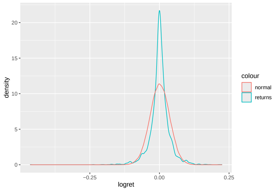
Figura 6.4: Densidad de rendimientos del Bitcoin Vs. una distribución normal
