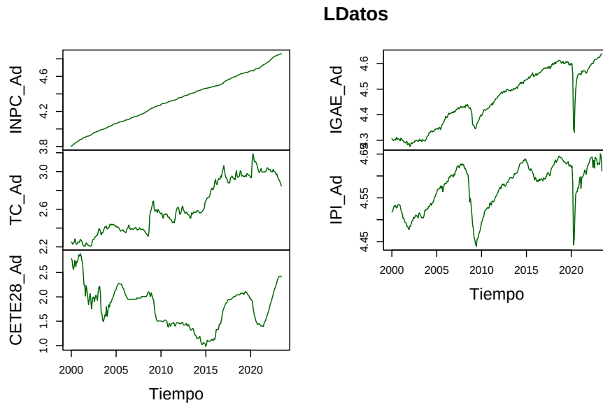
Figura 5.9: Series en niveles (logaritmos) para la prueba de Cointegración
