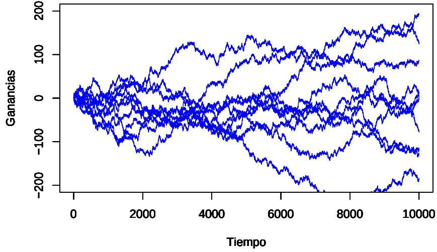
Figura 3.1: Ejemplo de 10 trayectorias de la caminata aleatoria, cuando sólo son posibles cambios de +1 y -1
