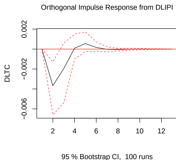
Figura 5.8: Impulso - Respuesta en DLTC_t
