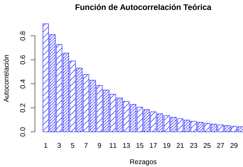
Figura 3.7: Función de Autocorrelación Teórica
