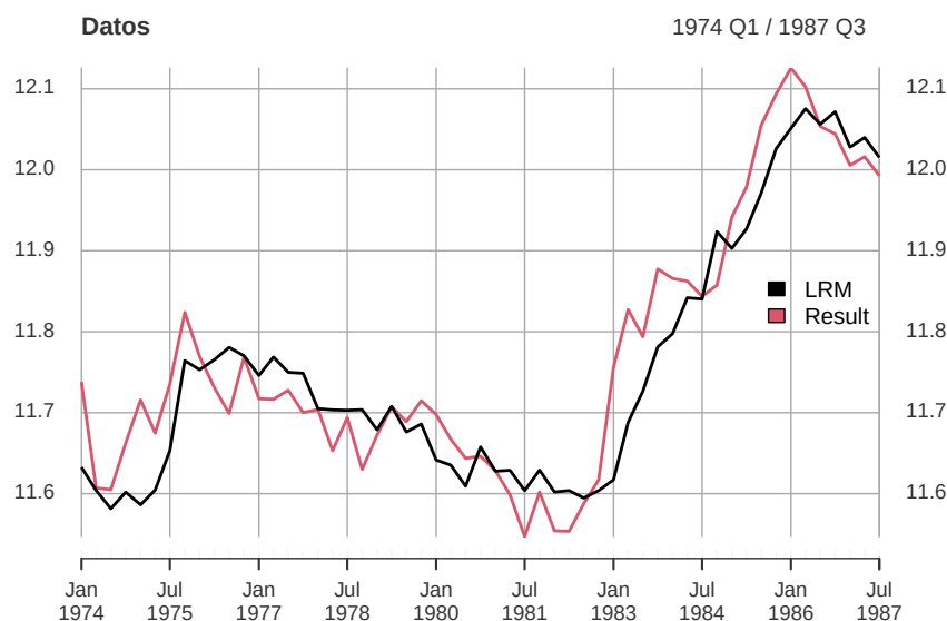
Figura 5.14: Gráfica de la ecuación de cointegración
