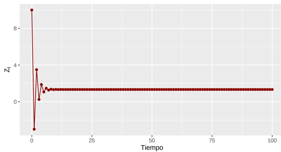
Figura 2.7: Evolución del proceso dado por Z_t = 2 - 0.5Z_{t-1}
