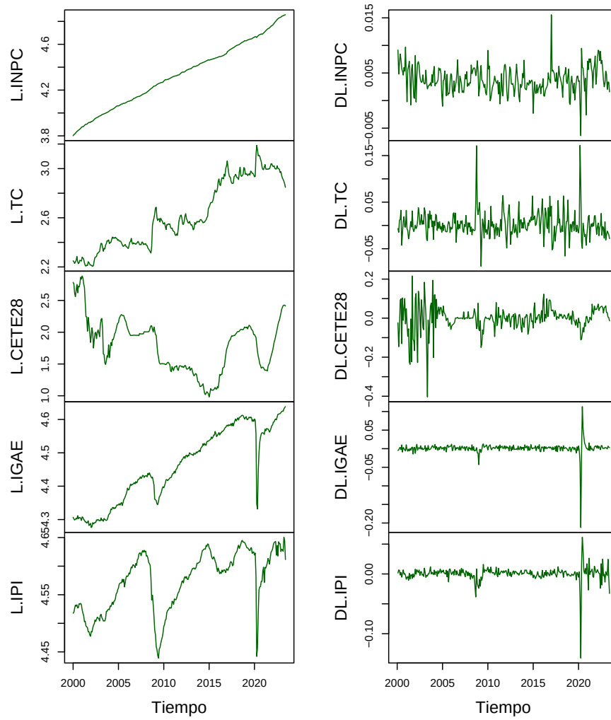
Figura 4.6: Comparación de Series en Niveles (Logaritmos) y en Diferencias Logarítmicas
