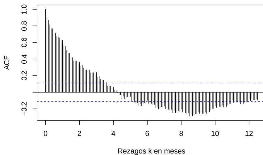
Figura 3.3: Función de Autocorrelación: 150 rezagos del número de pasajeros en el Metro de la CDMX, enero de 2000 a junio de 2025
