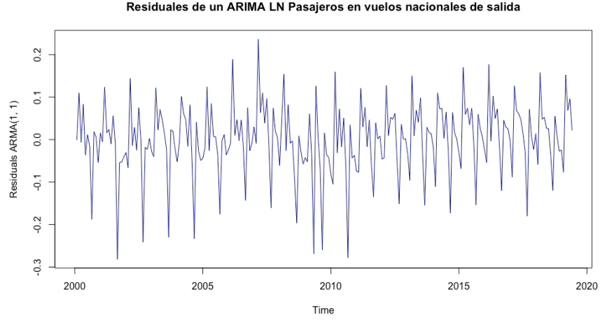
Figura 3.16: Residuales de un ARMA(1, 1) de la serie DLPaxNal_t
