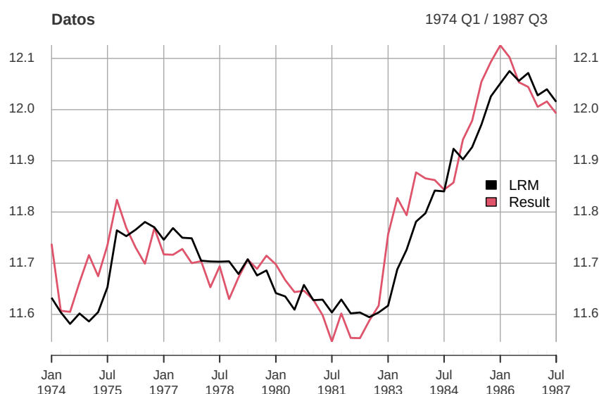
Figura 5.14: Gráfica de la ecuación de cointegración
