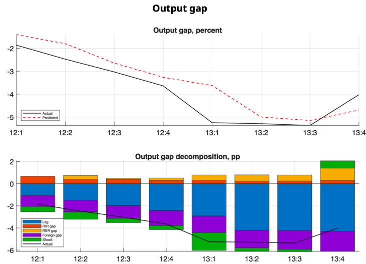
Figura 5.16: Simulación de la Descomposición de la Brecha del Producto. Elaboración propia con datos de IMF [-@imf2020].
