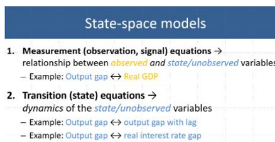
Figura 5.15: State-space models. Recuperado de IMF [-@imf2020].
