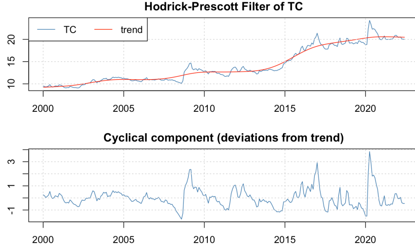
Figura 3.23: Descomposición del Tipo de Cambio FIX ( TC_t ) en su tendencia o trayectoria de largo plazo y su ciclo de corto plazo utilizando un filtro Hodrick y Prescott [-@hodrickprescott1997]
