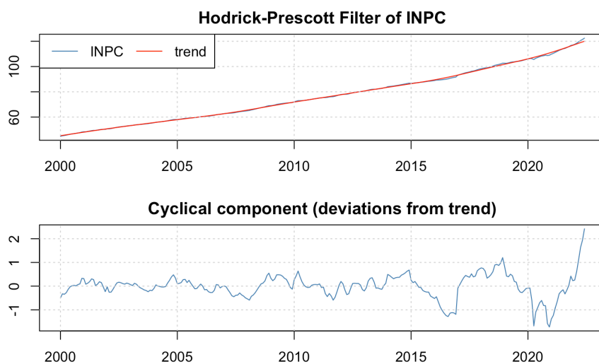
Figura 3.22: Descomposición del Índice Nacional de Precios al Consumidor ( INPC_t ) en su tendencia o trayectoria de largo plazo y su ciclo de corto plazo utilizando un filtro Hodrick y Prescott [-@hodrickprescott1997]
