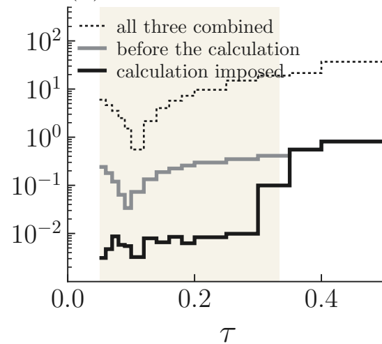
(d) learning
