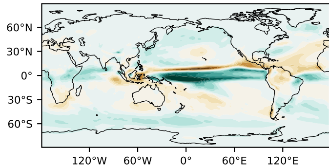
CMIP6
