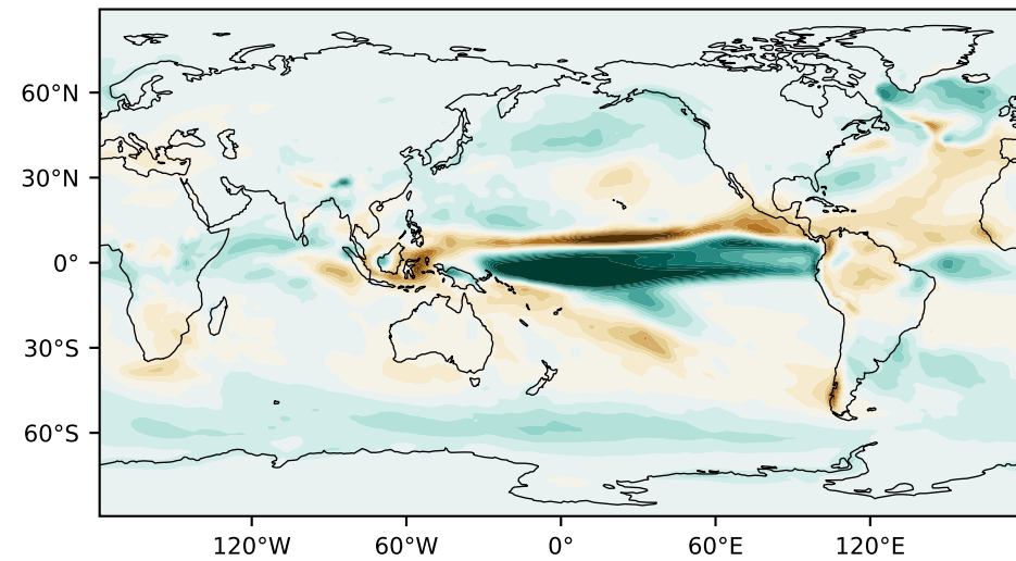
CESM2-WACCM
