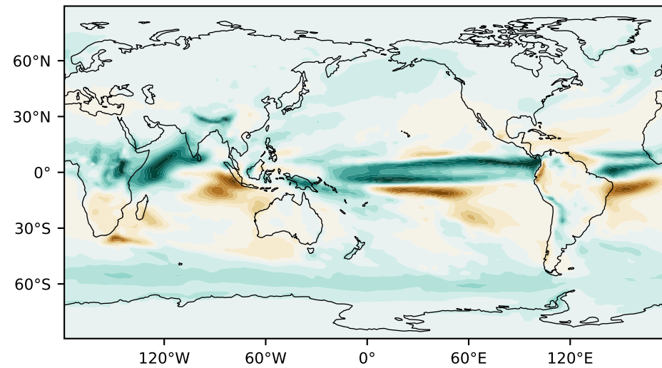
CMCC-ESM2
