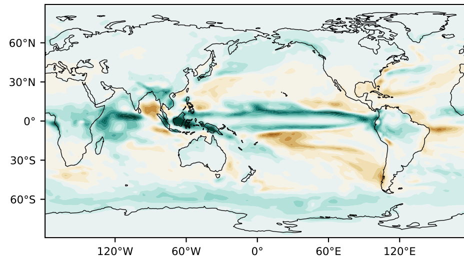
MIROC-ES2L
