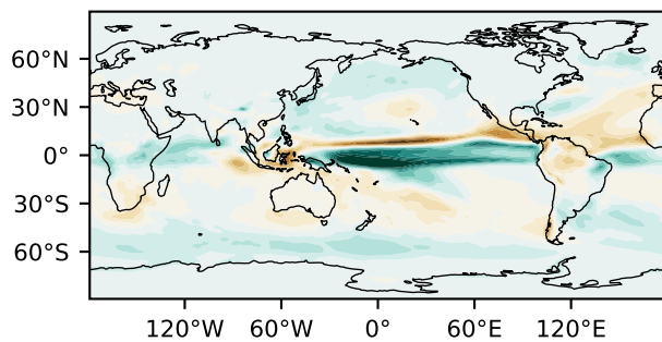
b CMIP6
