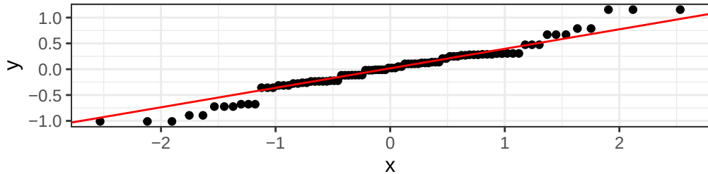
Normal Q-Q
