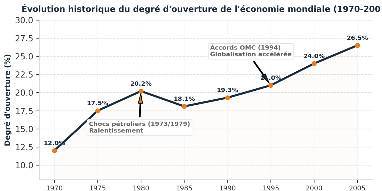
Graphique 2 : Évolution historique du taux d'ouverture de l'économie mondiale depuis 1970.
