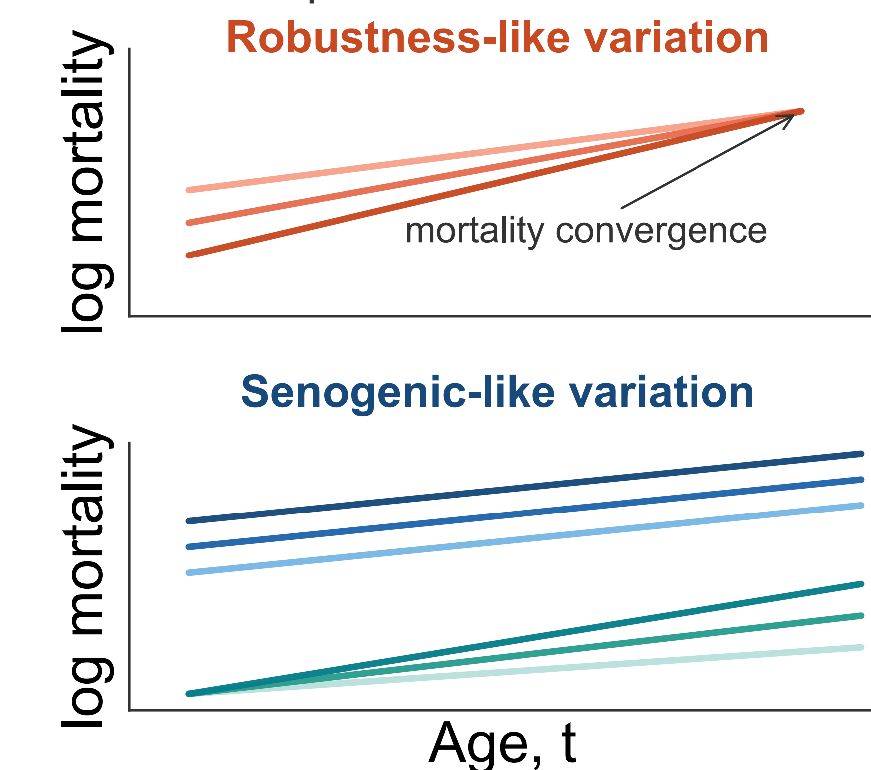
d Mortality signatures of parameter classes
