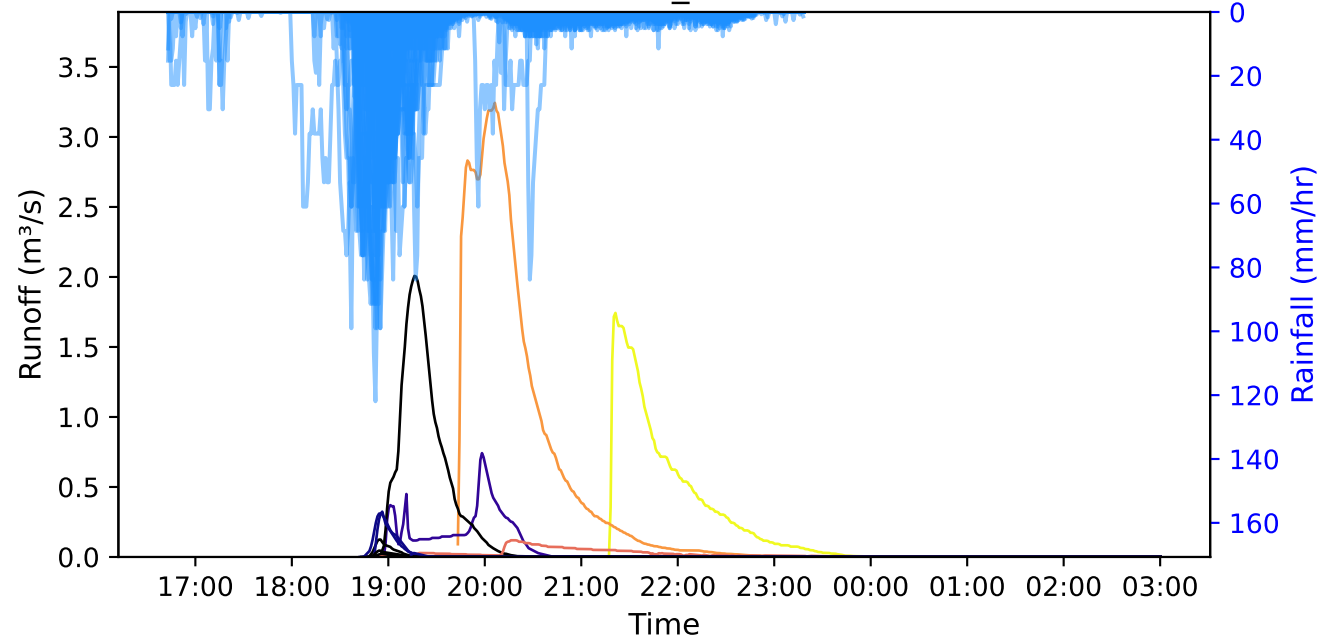
event_201
