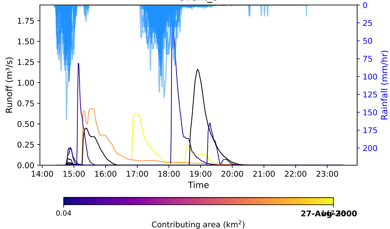
event_9
