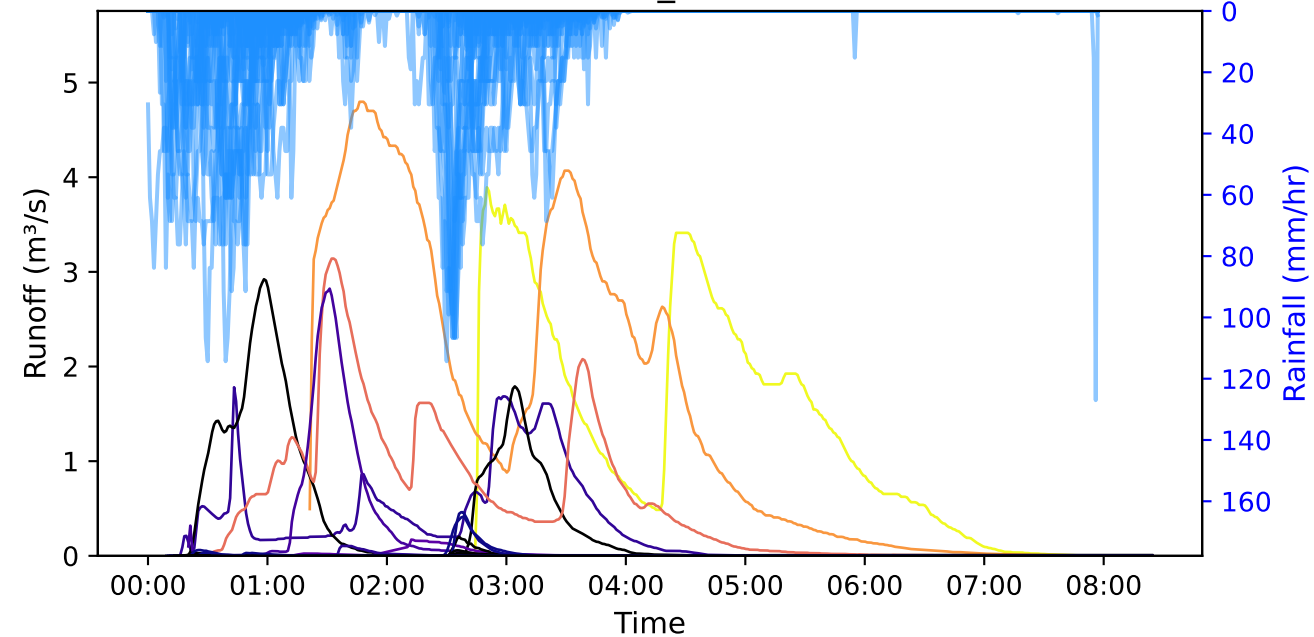
event_202
