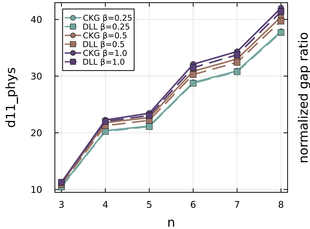
(b) d_{\{1 \rightarrow 1\}} vs n — CKG \approx DLL
