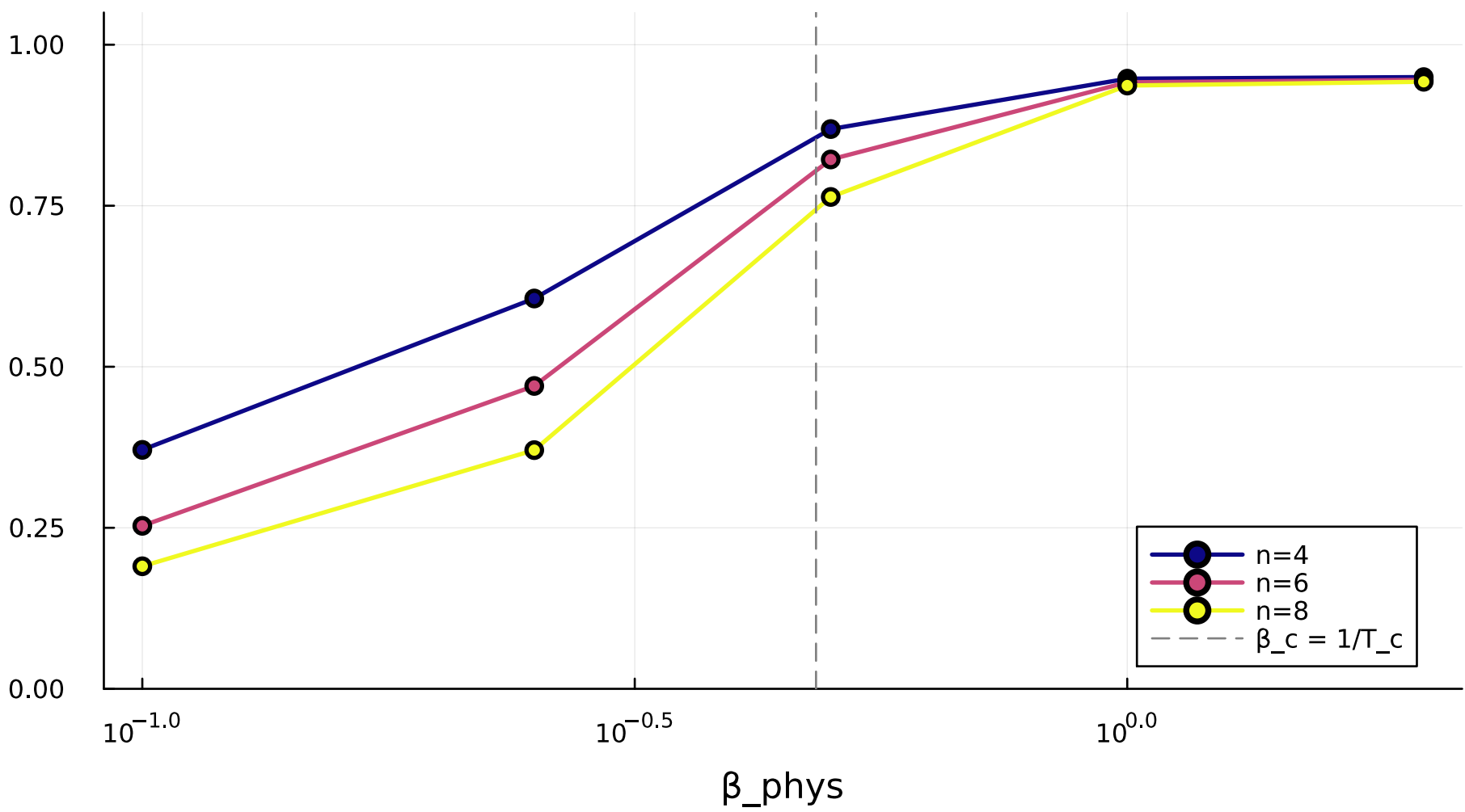
(b) Binder cumulant
