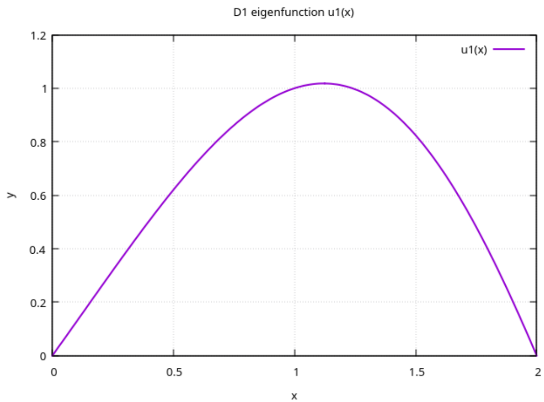
Рис. 6 Собственная функций для числа 5.16796
