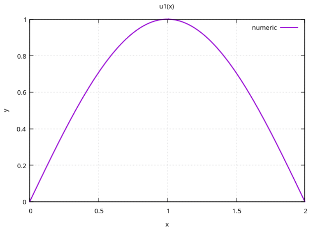
Рис. 4 Собственная функций для числа 2.4674
