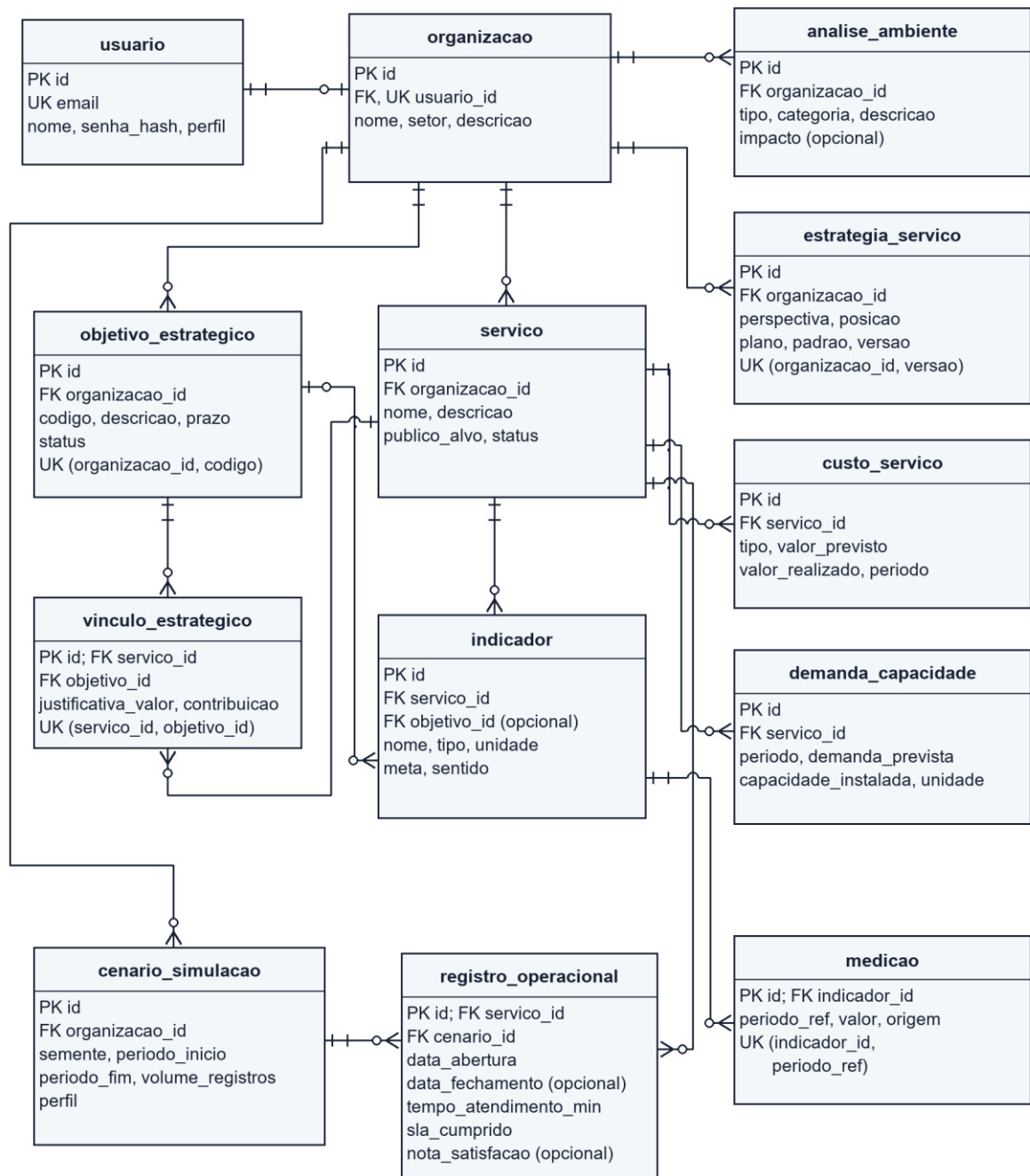
Imagem 7 - Modelo lógico relacional em notação pé de galinha
