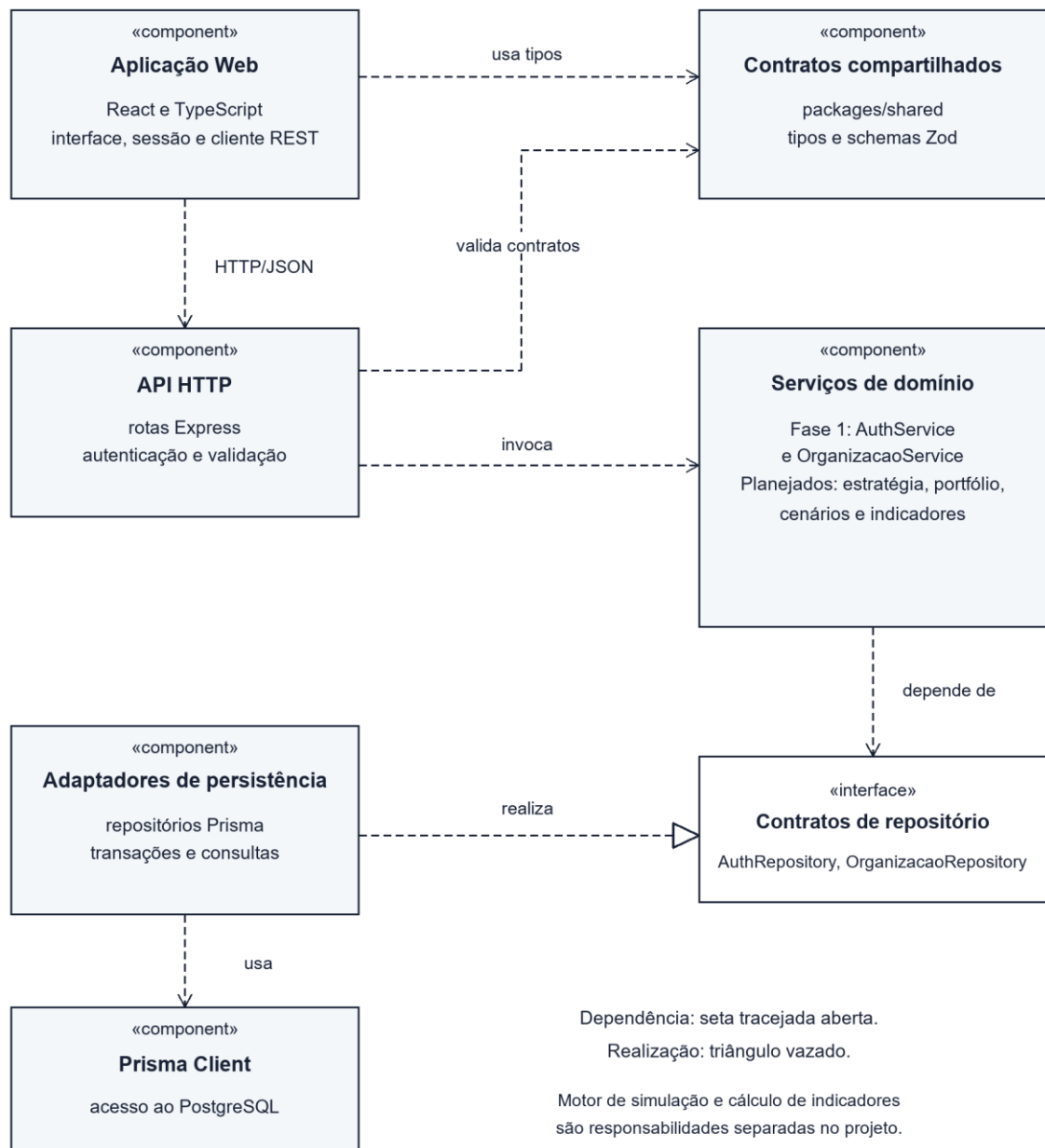
Imagem 8 - Diagrama de componentes UML da solução
