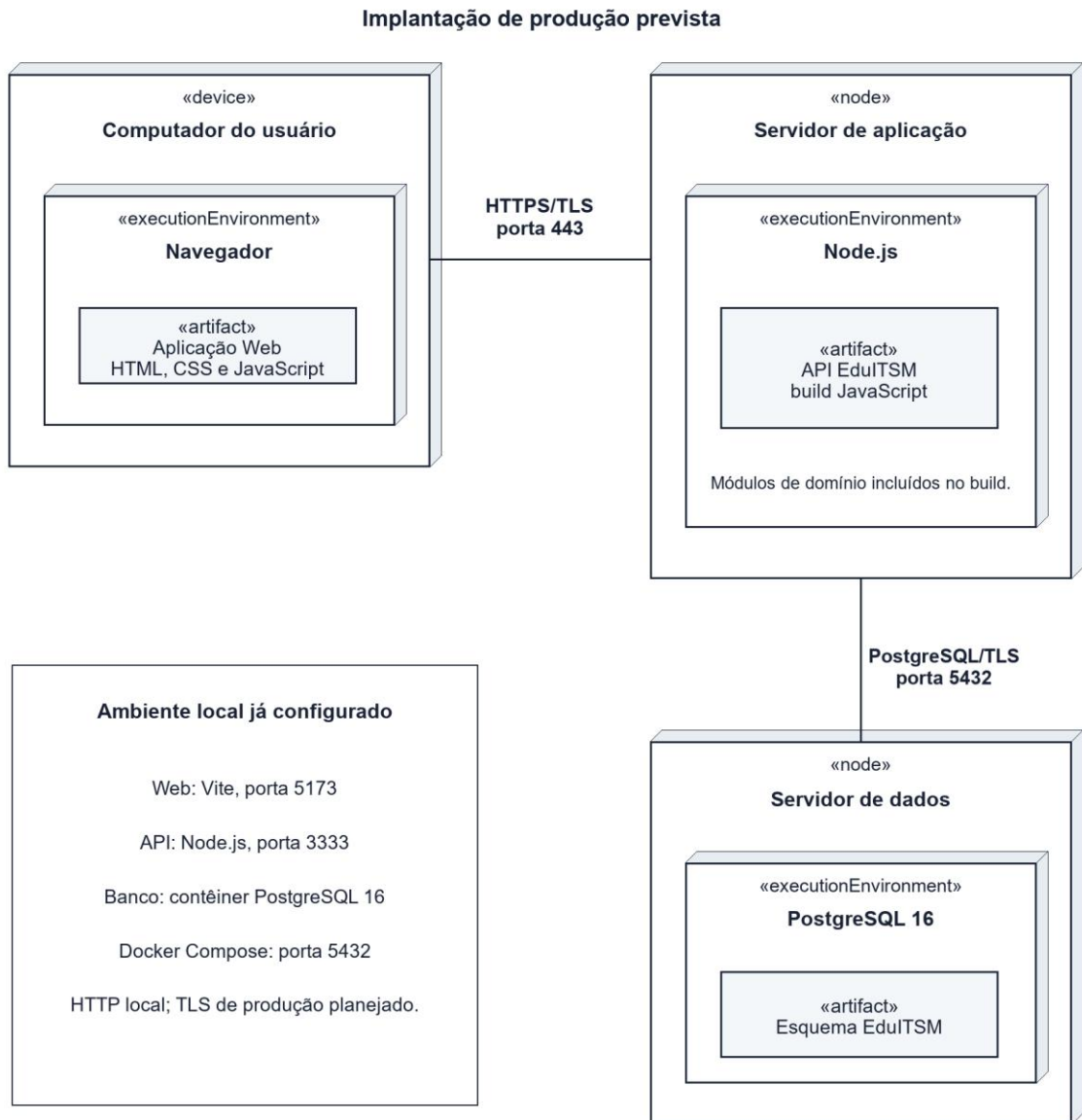
Imagem 9 - Diagrama de implantação UML da solução
