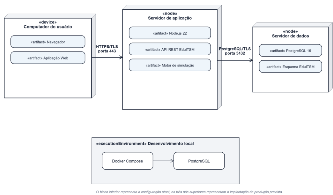
Imagem 9 - Diagrama de implantação UML da solução
