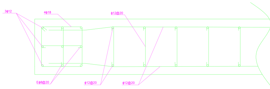
Figura 3.2: Esquema de muros con resumen de armadura de corte y flexo-compresión. Piso 1.
