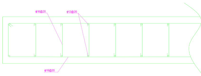
Figura 3.3: Esquema de muros con resumen de armadura de corte y flexo-compresión. Piso 2.
