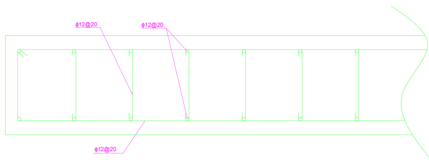
Figura 3.4: Esquema de muros con resumen de armadura de corte y flexo-compresión. Piso 3.
