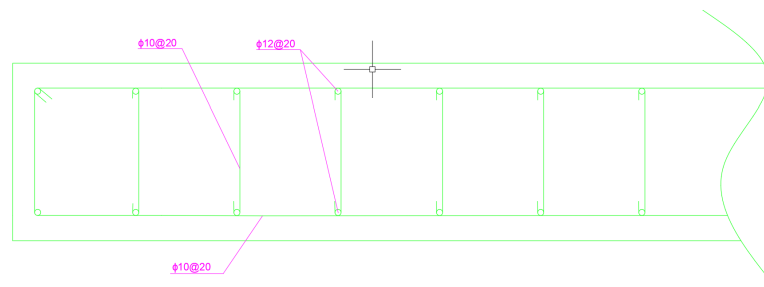
Figura 3.5: Esquema de muros con resumen de armadura de corte y flexo-compresión. Pisos 5, 8, 11 y 15.
