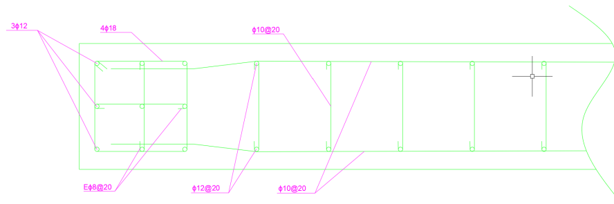
Figura 3.1: Esquema de muros con resumen de armadura de corte y flexo-compresión. Piso -1.
