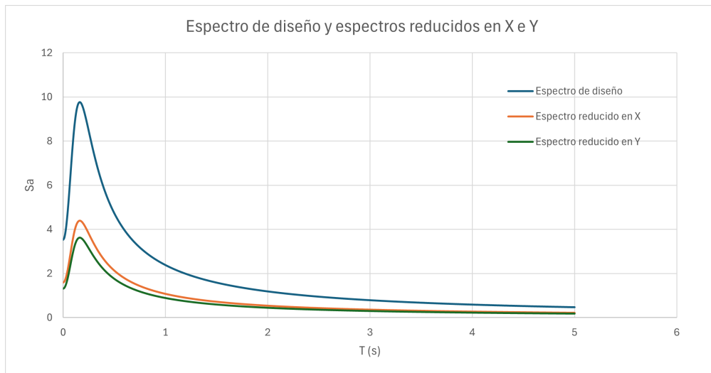
Figura 1: Espectro elástico y espectros reducidos para las direcciones X e Y, según NCh433 Instituto Nacional de Normalización (2009).
