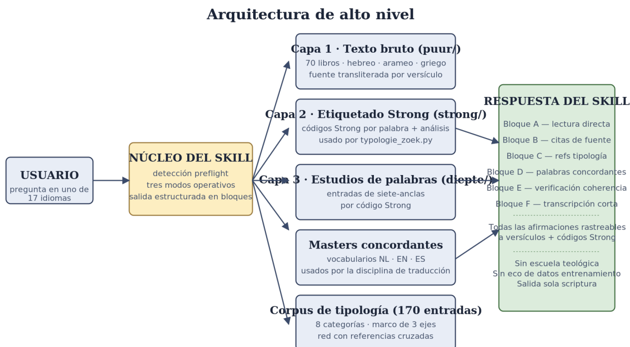
Figura 1 — Diagrama de componentes de alto nivel. El skill nunca sirve respuestas desde la memoria de entrenamiento; cada bloque alcanza el corpus.
